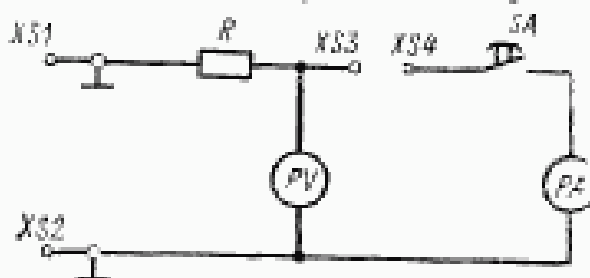
РА—амперметр; PV—вольтметр.
