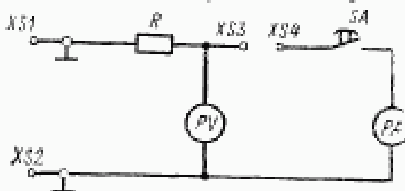
РА—амперметр; PV—вольтметр.
