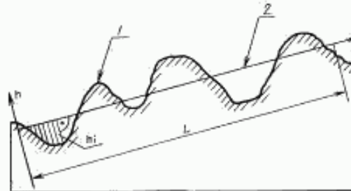
1 — реальный профиль; 2 — средняя прямая
