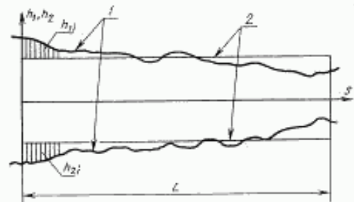
1 — реальный профиль; 2 — средний профиль продольного сечения
