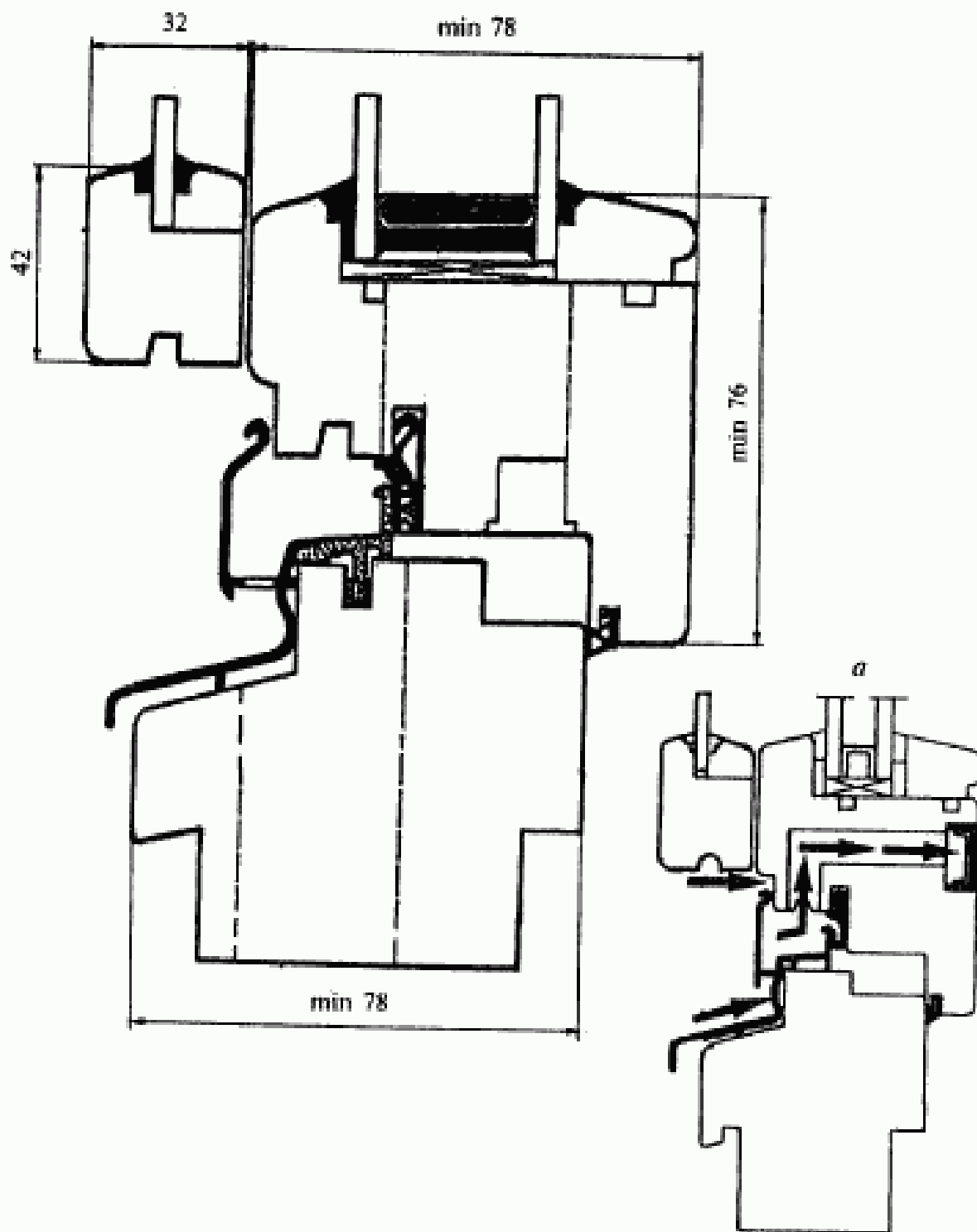
a — вариант установки климатического клапана
