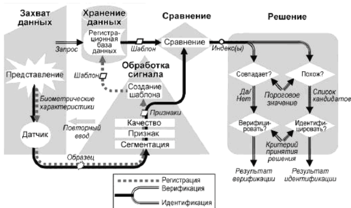
Рисунок 1 – Компоненты унифицированной биометрической системы
