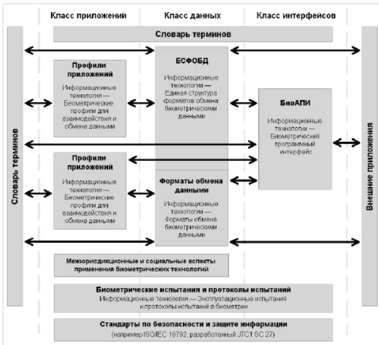
Рисунок 4 – Взаимосвязь базовых биометрических стандартов
