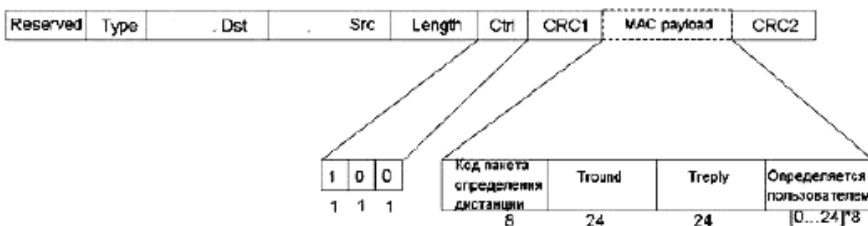
Рисунок 51 – Формат пакета измерения расстояния T2R3
