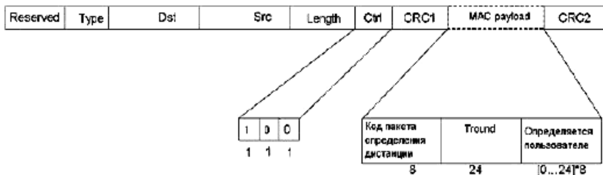
Рисунок 55 – Формат пакета измерения расстояния T4R2
