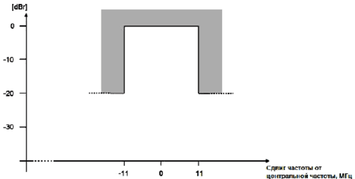
Рисунок 6 – Пределы передаваемой СПМ для двухточечной ортогональной ЛЧМ с полосой частот 22 МГц
