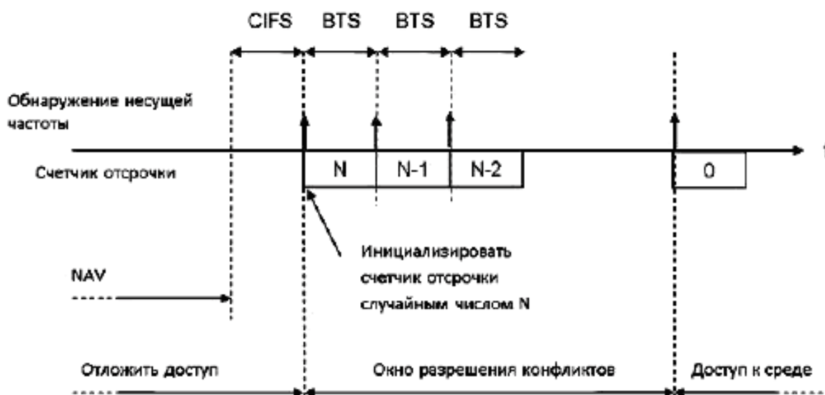
Рисунок 27 – Процедура отсрочки передачи с CSMA/CA
