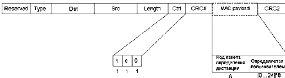
Рисунок 49 – Формат пакета измерения расстояния T2R1
