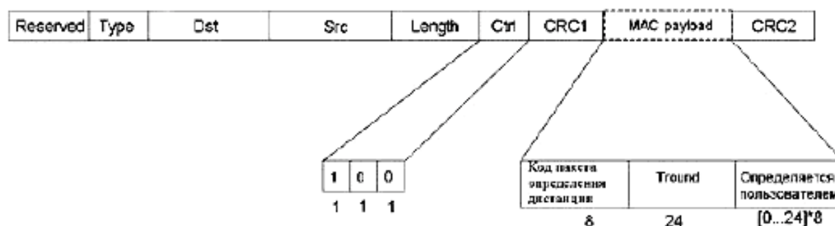
Рисунок 48 – Формат пакета измерения расстояния T1R3
