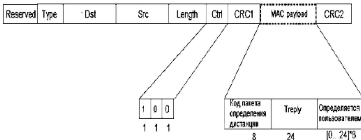
Рисунок 47 – Формат пакета измерения расстояния T1R2
