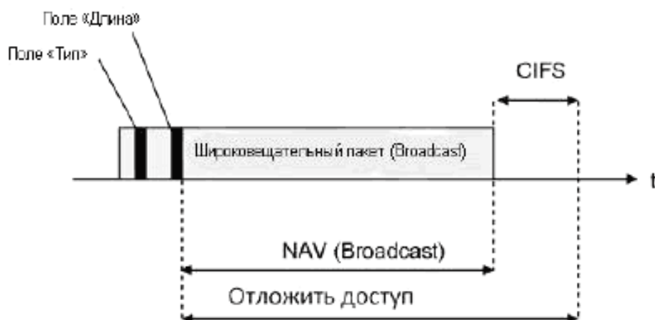
Рисунок 25 – NAV для пакетов «Широковещательный пакет» (Broadcast)
