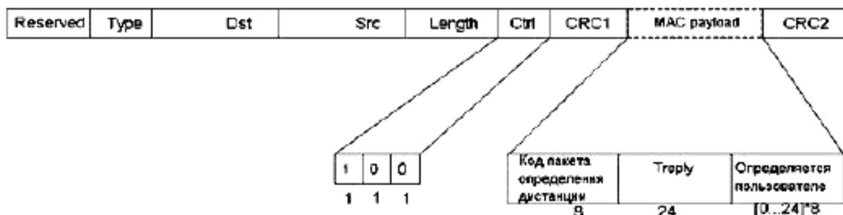
Рисунок 53 – Формат пакета измерения расстояния T3R2
