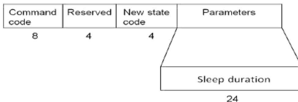
Рисунок 35 – Формат команды «Переключение в состояние «Энергосбережение» (SwitchState(Sleep))
