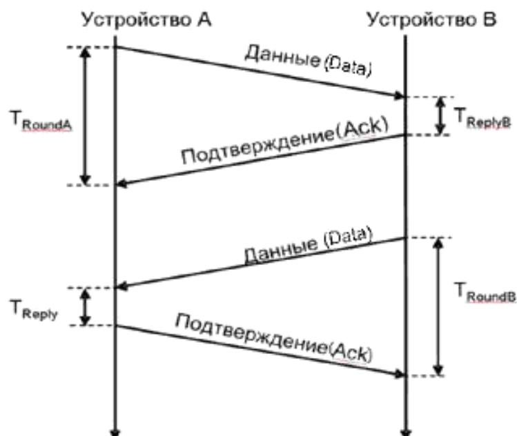
Рисунок А.2 – Метод СДС-ДНОД при обмене пакетами данных с подтверждением
