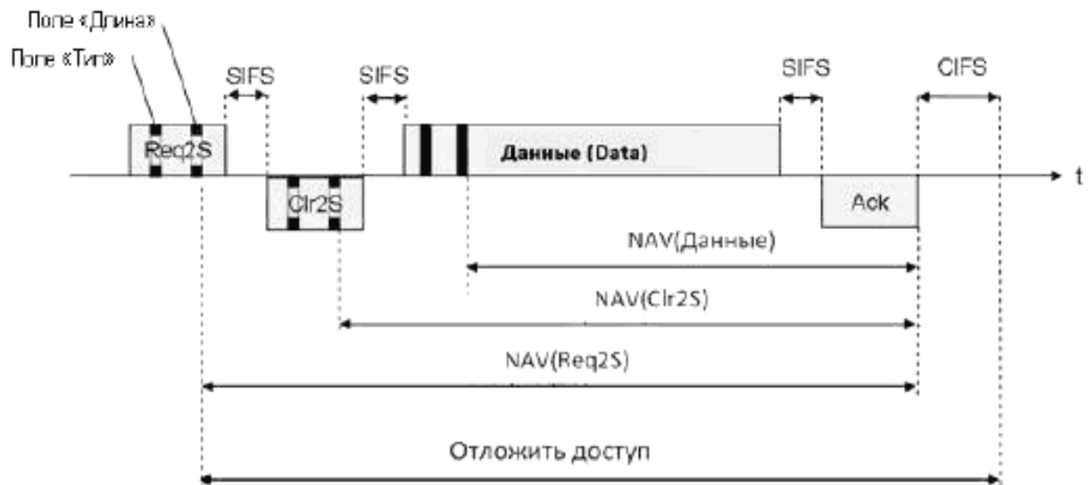
Рисунок 26 – NAV для трехэтапного установления связи
