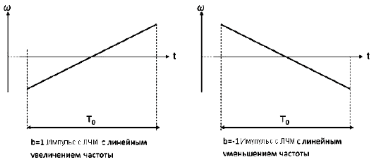
Рисунок 9 – Импульсы с ЛЧМ в частотно-временной области
