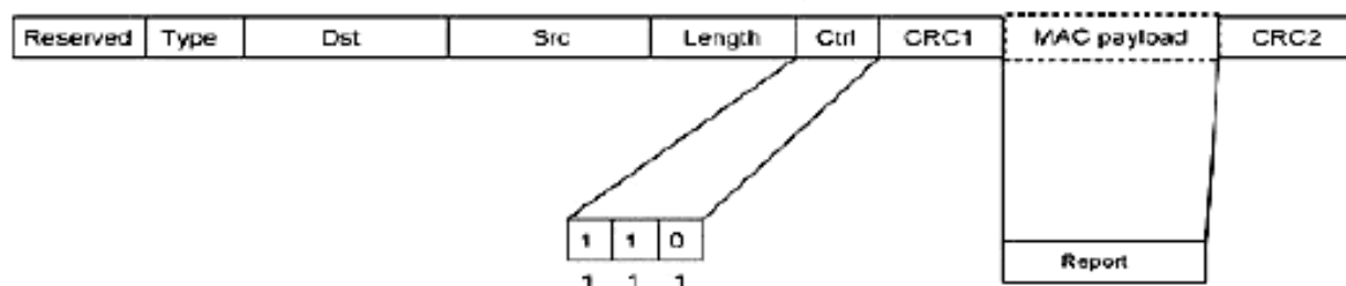
Рисунок 42 – Формат прикладных пакетов отчетов
