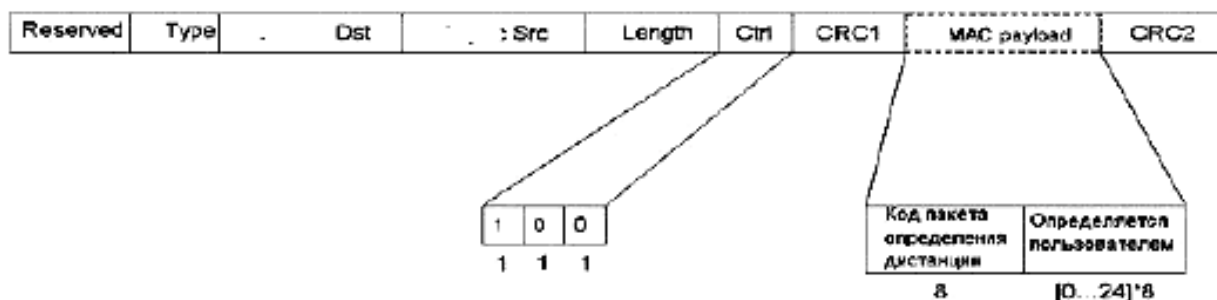
Рисунок 54 – Формат пакета измерения расстояния T4R1
