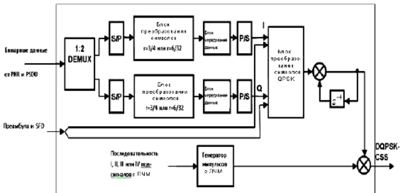
Рисунок 12 – Эталонный модулятор для DQPSK-CSS
