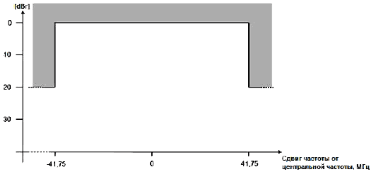
Рисунок 5 – Пределы передаваемой СПМ для двухточечной ортогональной ЛЧМ с полосой частот 80 МГц
