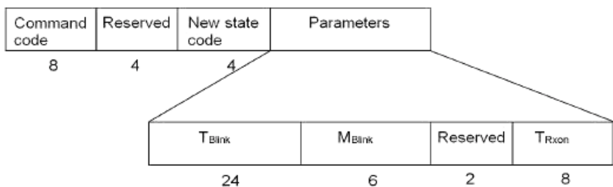
Рисунок 32 – Формат команды «Переключение в состояние «Передача блинк-посылки» (SwitchState(Blink))
