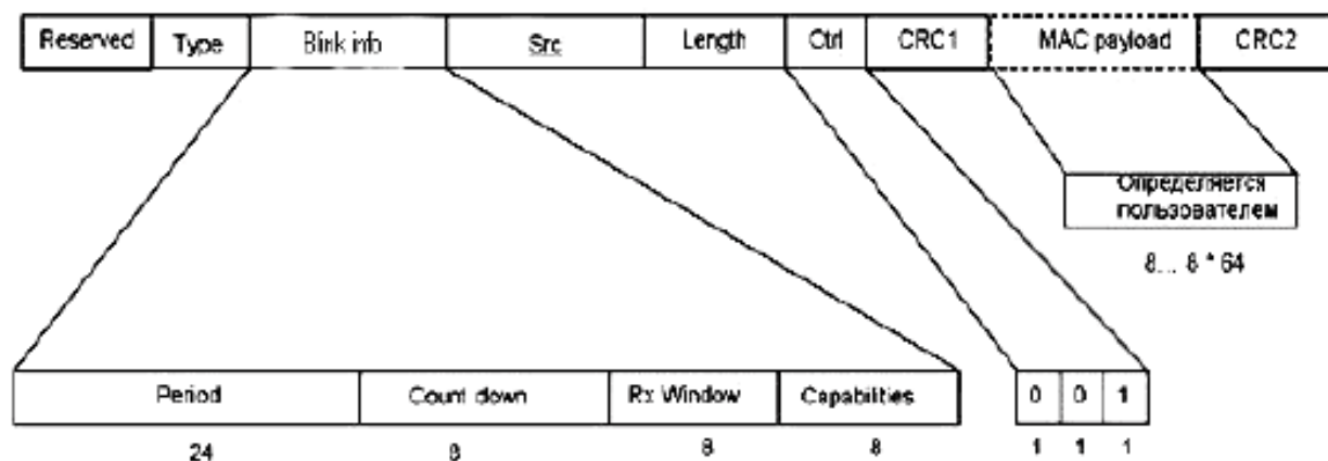
Рисунок 40 – Формат прикладного пакета передачи блинк-посылки
