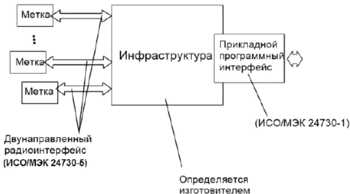
Рисунок 1 – Составные части системы RTLS
