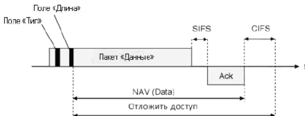
Рисунок 24 – NAV для пакетов «Данные» (Data)
