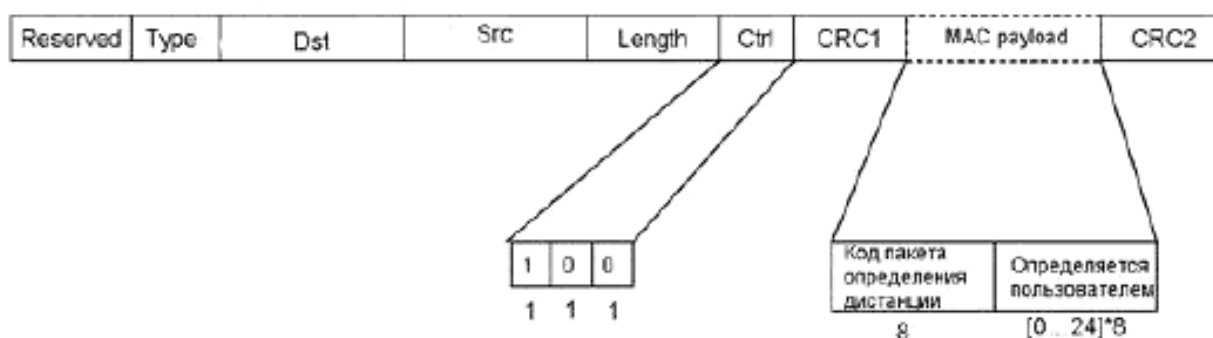
Рисунок 46 – Формат пакета измерения расстояния T1R1
