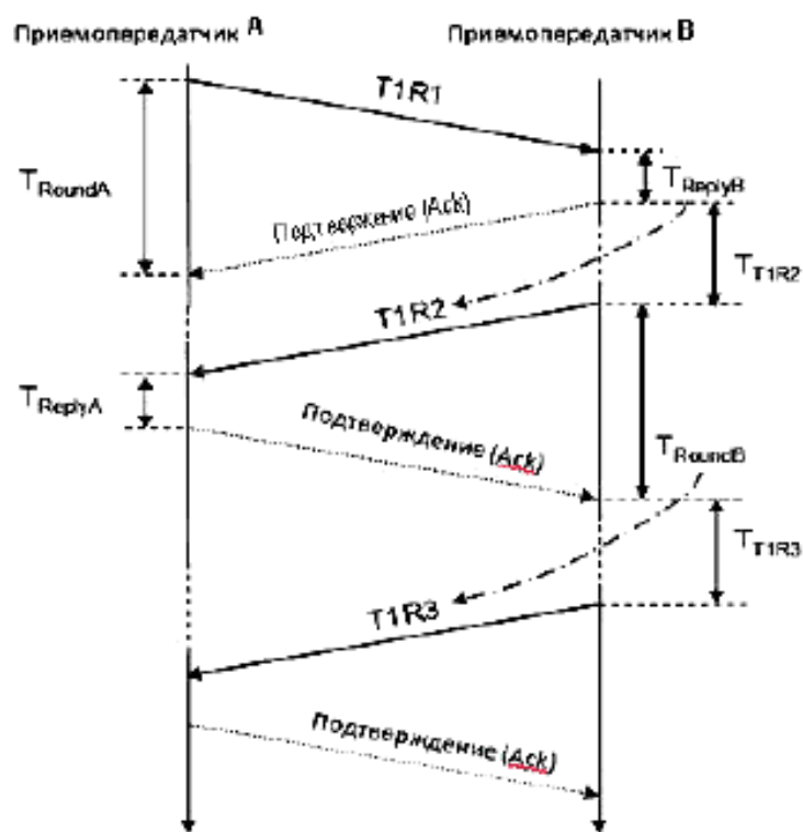
Рисунок 56 – Обмен пакетами измерения расстояния типа 1
