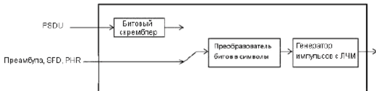
Рисунок 4 – Эталонный модулятор для двухточечной ортогональной ЛЧМ
