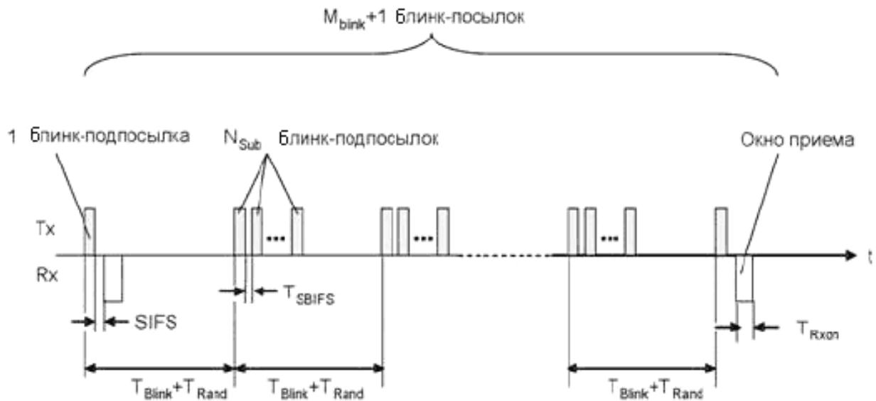
Рисунок 29 – Режим передачи блинк-посылки
