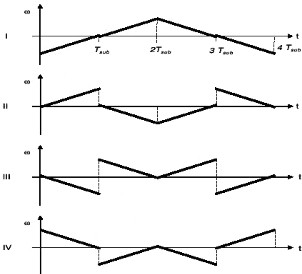
Рисунок 14 – Четыре последовательности подсигналов с ЛЧМ
