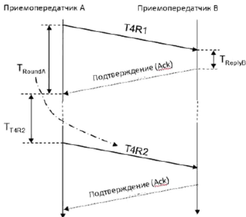
Рисунок 59 – Обмен пакетами измерения расстояния типа 4
