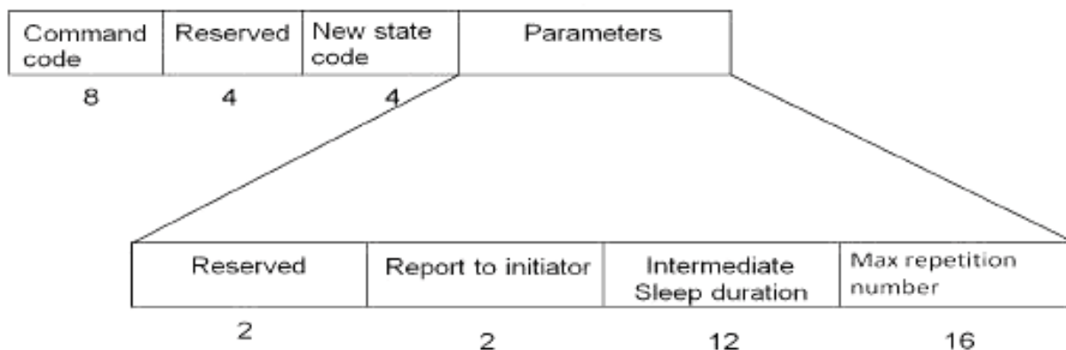
Рисунок 34 – Формат команды «Переключение в состояние «Измерение расстояния» (SwitchState(Range))
