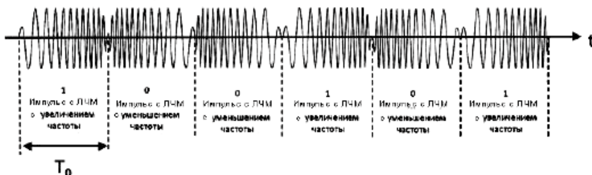
Рисунок 10 – Модулированная двоичная последовательность двухточечной ортогональной ЛЧМ
