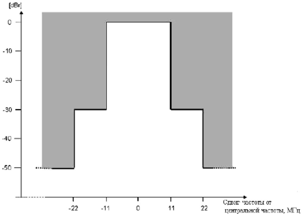
Рисунок 13 – Диапазон для передаваемой СПМ в случае DQPSK-CSS
