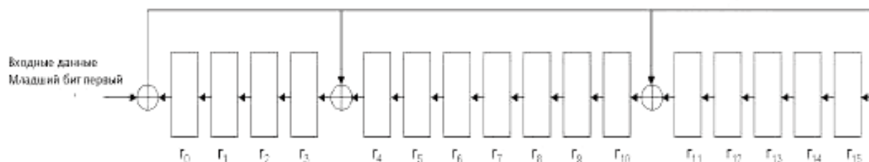
Рисунок 21 – Вычисление значения циклического избыточного кода (CRC) с помощью регистра LFSR
