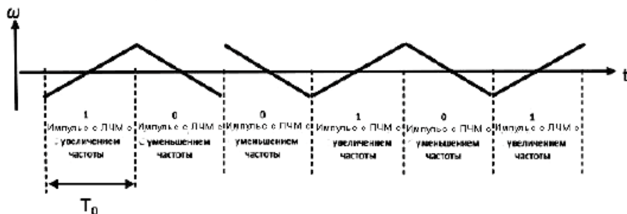
Рисунок 11 – Модулированная двоичная последовательность двухточечной ортогональной ЛЧМ в частотно-временной области
