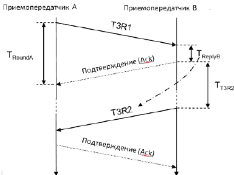
Рисунок 58 – Обмен пакетами измерения расстояния типа 3
