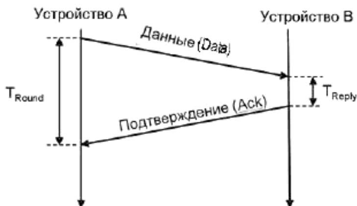
Рисунок А.1 – Двунаправленное измерение расстояния
