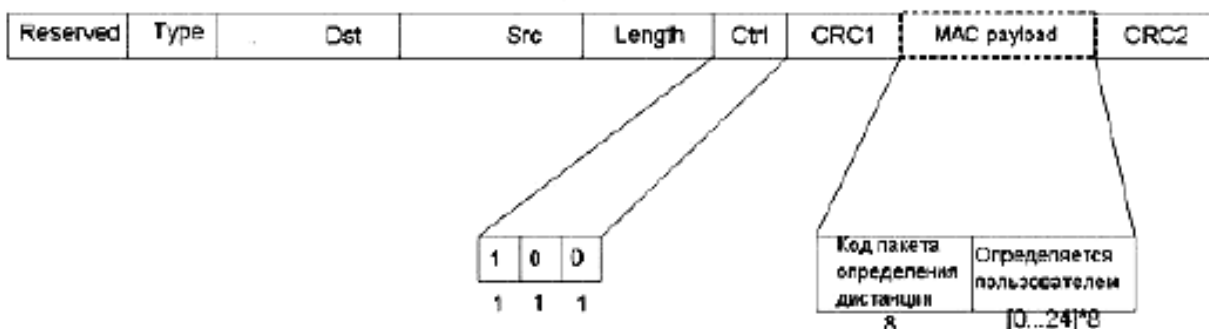
Рисунок 52 – Формат пакета измерения расстояния T3R1
