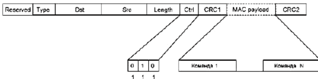
Рисунок 41 – Формат прикладного пакета команд
