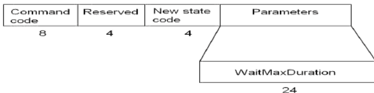
Рисунок 33 – Формат команды «Переключение в состояние «Ожидание» (SwitchState (Wait))
