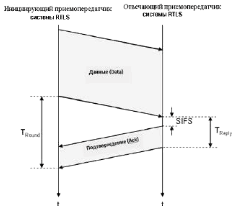
Рисунок 22 – Временные параметры подтверждения данных
