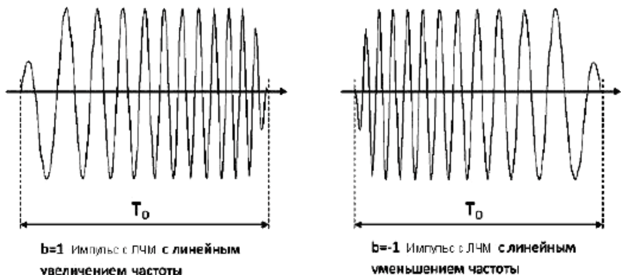
Рисунок 8 – Импульсы с ЛЧМ в полосе пропускания
