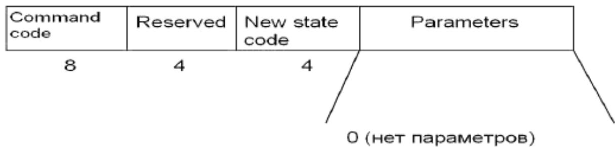
Рисунок 31 – Формат команды «Переключение в состояние «По умолчанию» (SwitchState(Default))
