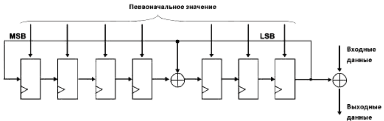
Рисунок 7 – Битовый скремблер (Bit scrambler)
