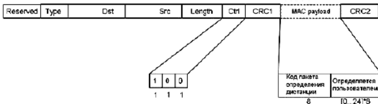
Рисунок 50 – Формат пакет измерения расстояния T2R2
