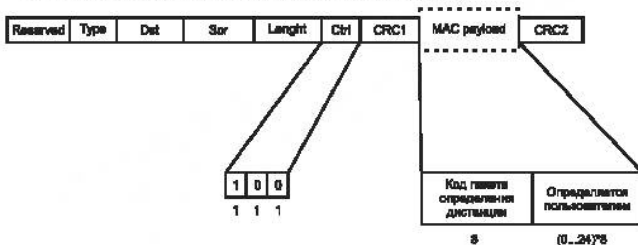
Рисунок 50 – Формат пакета измерения расстояния T2R2
