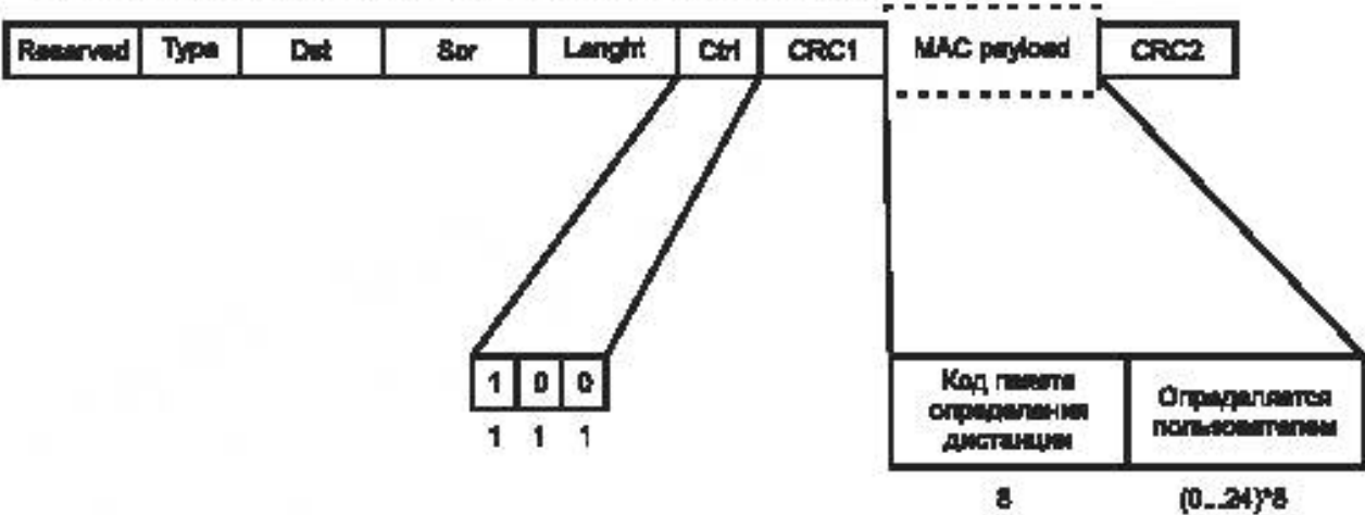
Рисунок 52 – Формат пакета измерения расстояния T3R1
