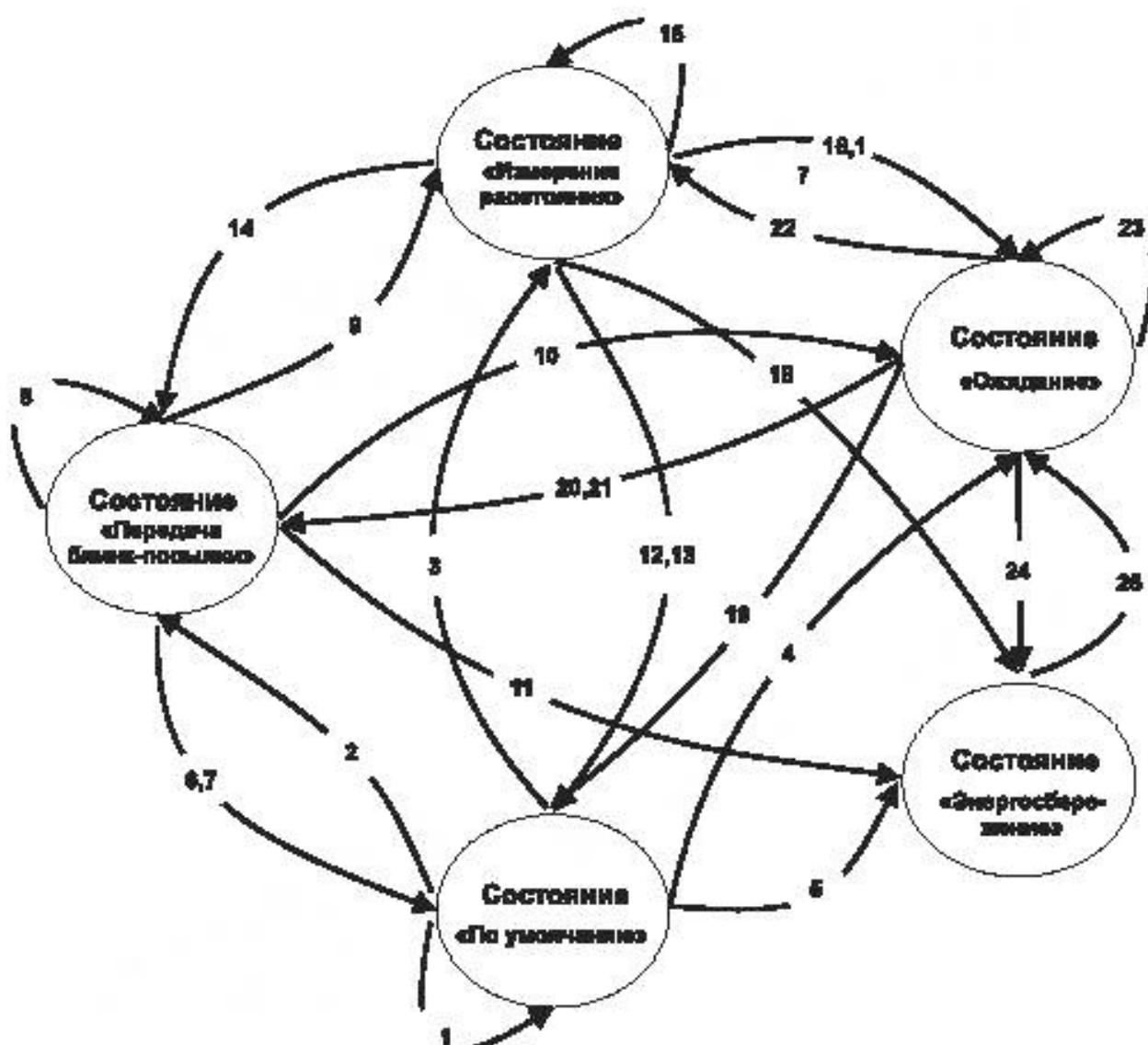
Рисунок 28 – Состояния метки на прикладном уровне
