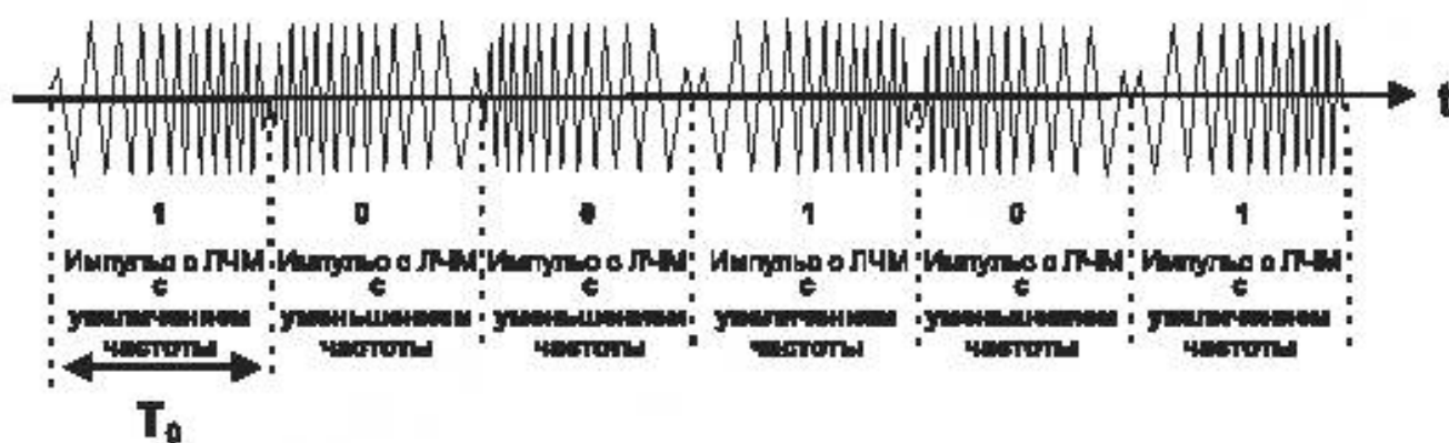
Рисунок 10 – Модулированная двоичная последовательность двухточечной ортогональной ЛЧМ
