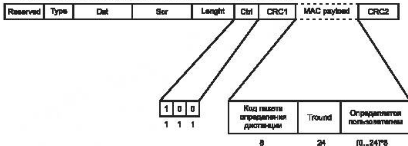
Рисунок 55 – Формат пакета измерения расстояния T4R2
