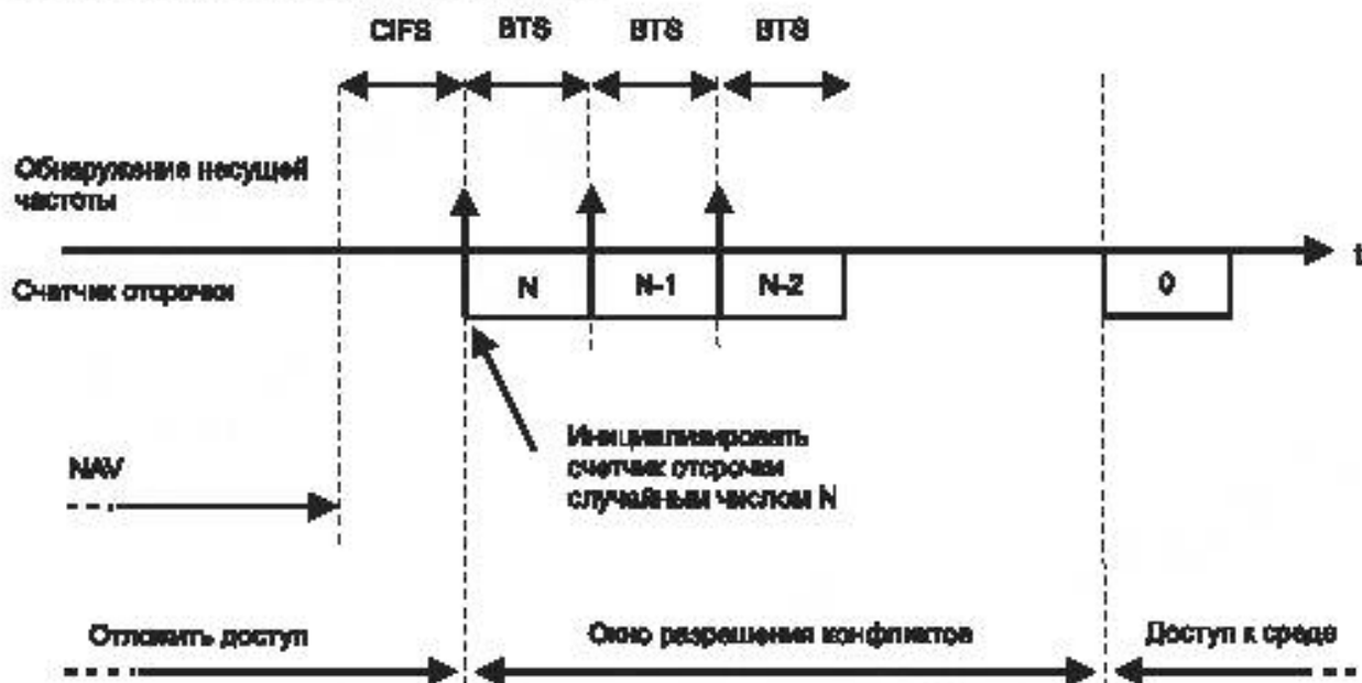
Рисунок 27 – Процедура отсрочки передачи с CSMA/CA
