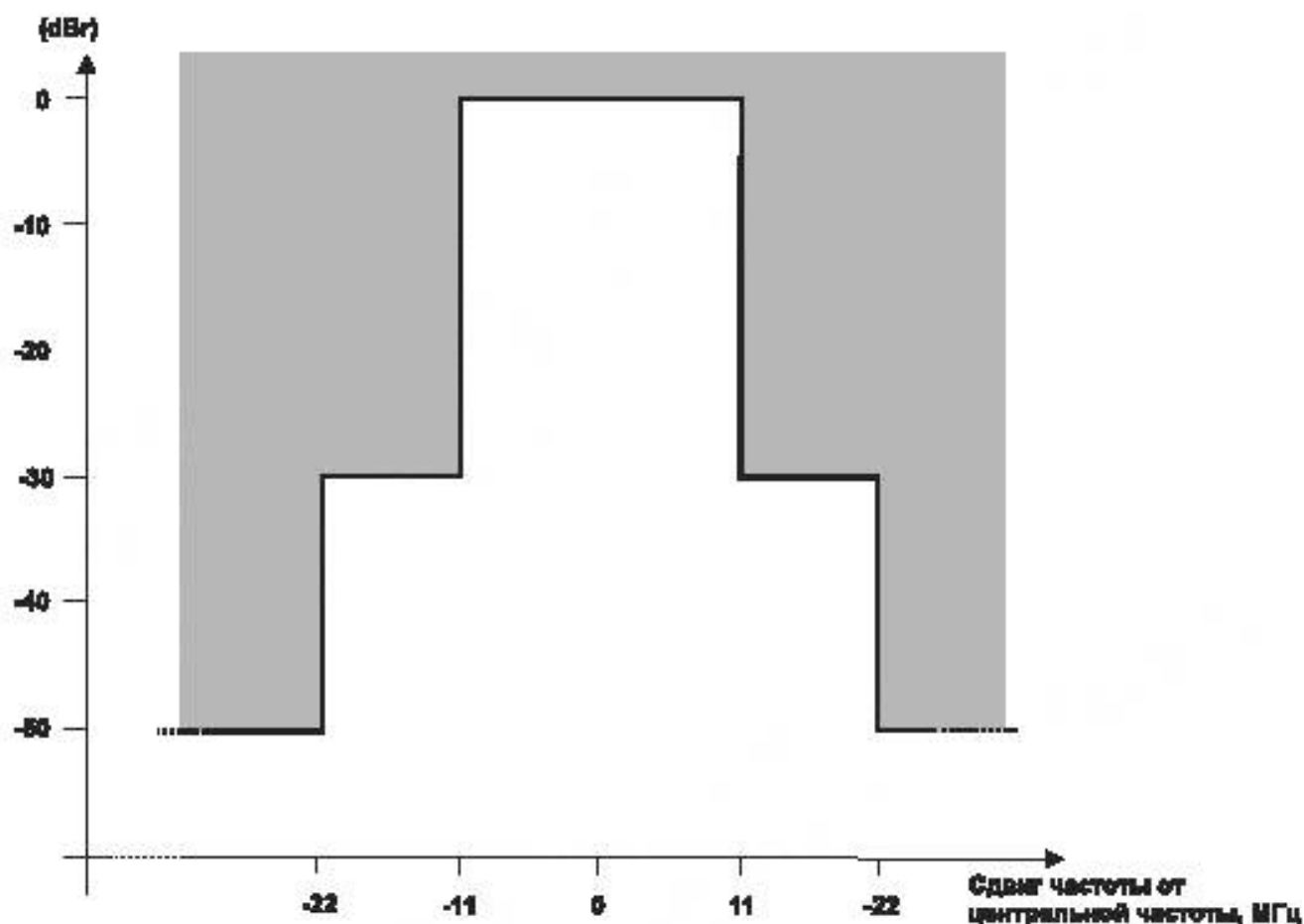
Рисунок 13 – Диапазон передаваемой СПМ в случае DQPSK-CSS
