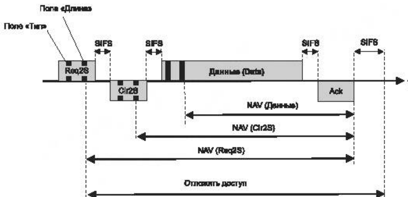
Рисунок 26 – NAV для трехэтапного установления связи
