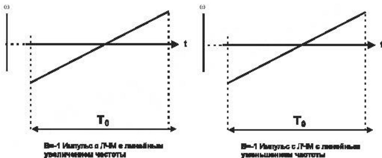
Рисунок 9 – Импульсы с ЛЧМ в частотно-временной области
