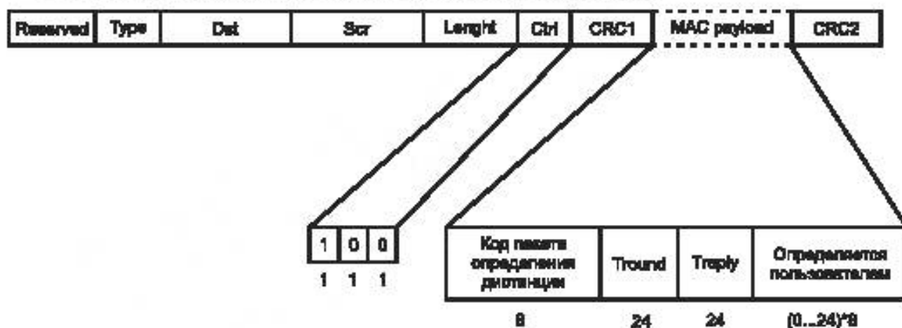
Рисунок 51 – Формат пакета измерения расстояния T2R3
