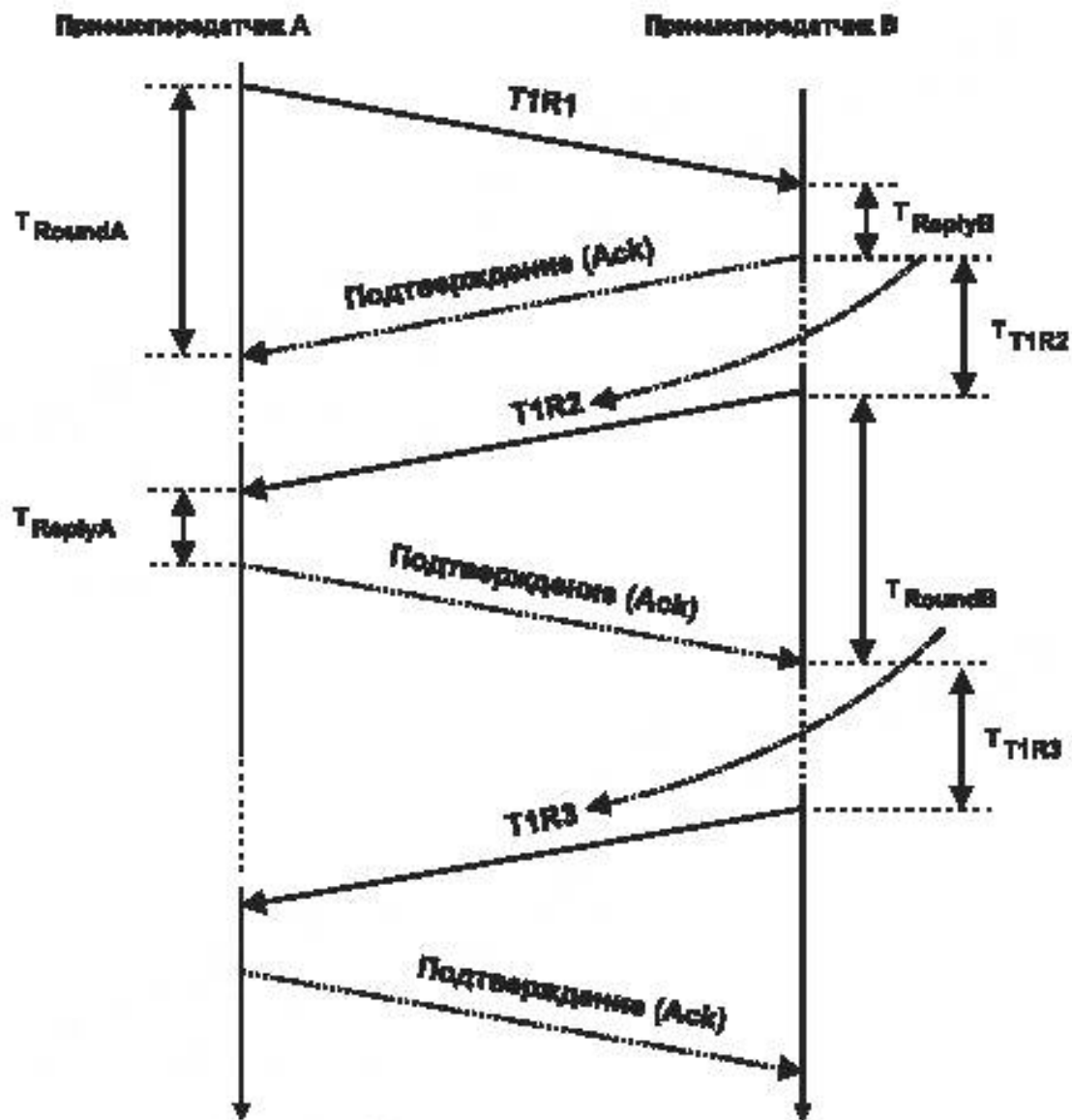
Рисунок 56 – Обмен пакетами измерения расстояния типа 1
