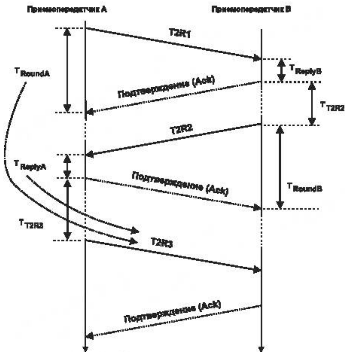
Рисунок 57 – Обмен пакетами измерения расстояния типа 2
