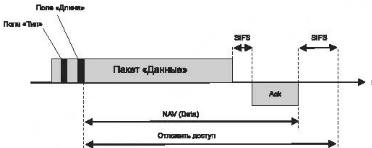
Рисунок 24 – NAV для пакетов «Данные» (Data)
