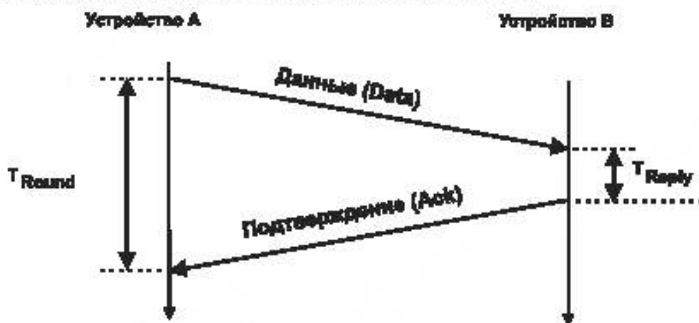
Рисунок А.1 – Двунаправленное измерение расстояния
