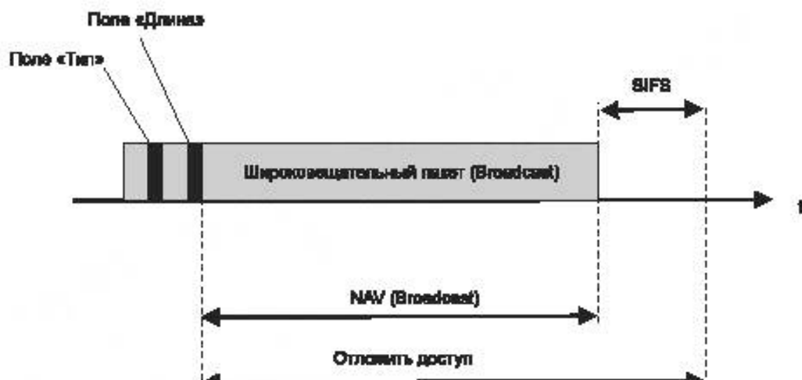
Рисунок 25 – NAV для пакетов «Широковещательный пакет» (Broadcast)
