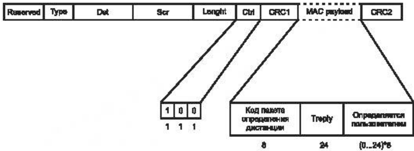
Рисунок 47 – Формат пакета измерения расстояния T1R2
