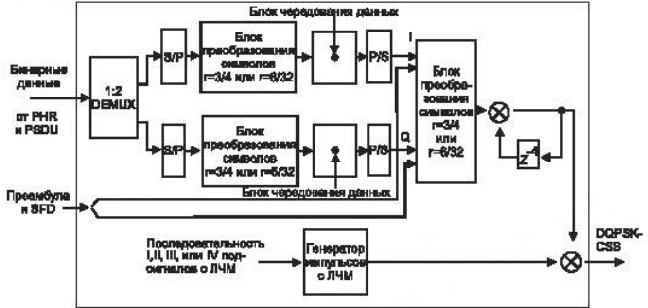
Рисунок 12 – Эталонный модулятор для DQPSK-CSS
