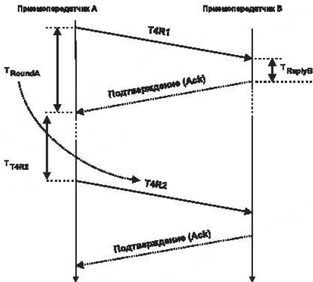
Рисунок 59 – Обмен пакетами измерения расстояния типа 4
