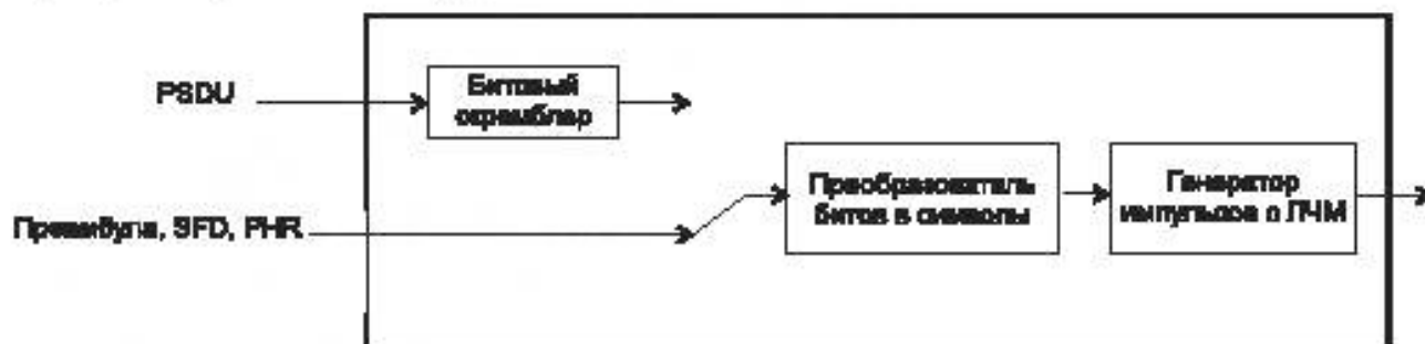
Рисунок 4 – Эталонный модулятор для двухточечной ортогональной ЛЧМ
