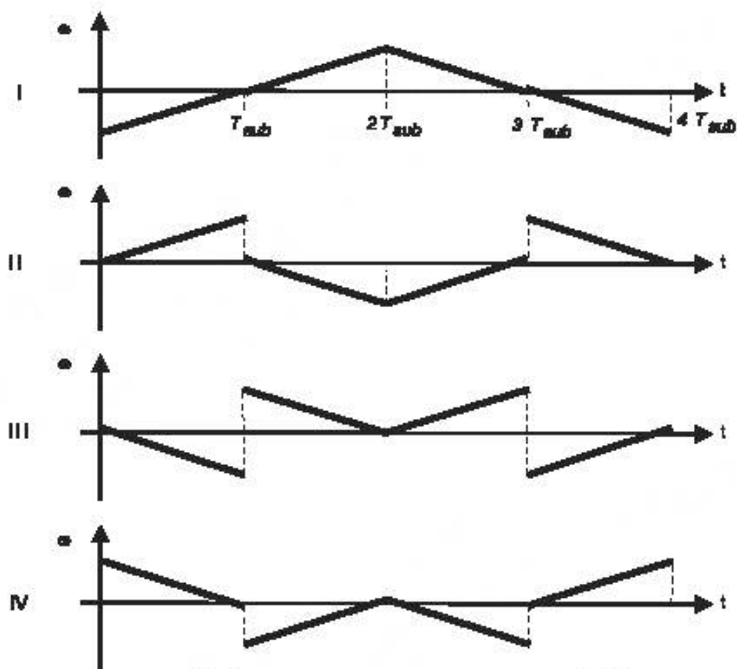
Рисунок 14 – Четыре последовательности подсигналов с ЛЧМ
