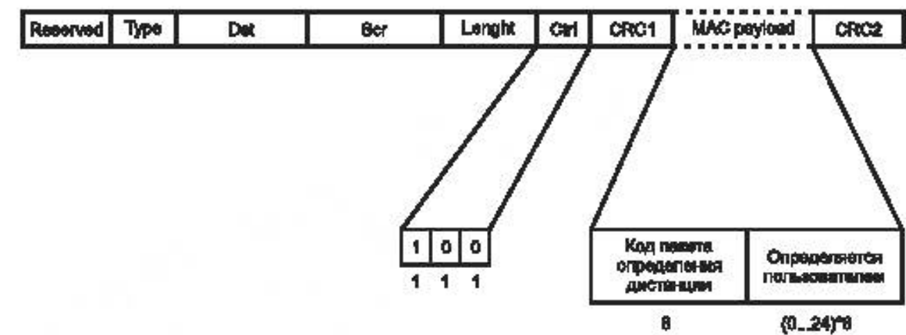
Рисунок 46 – Формат пакета измерения расстояния T1R1
