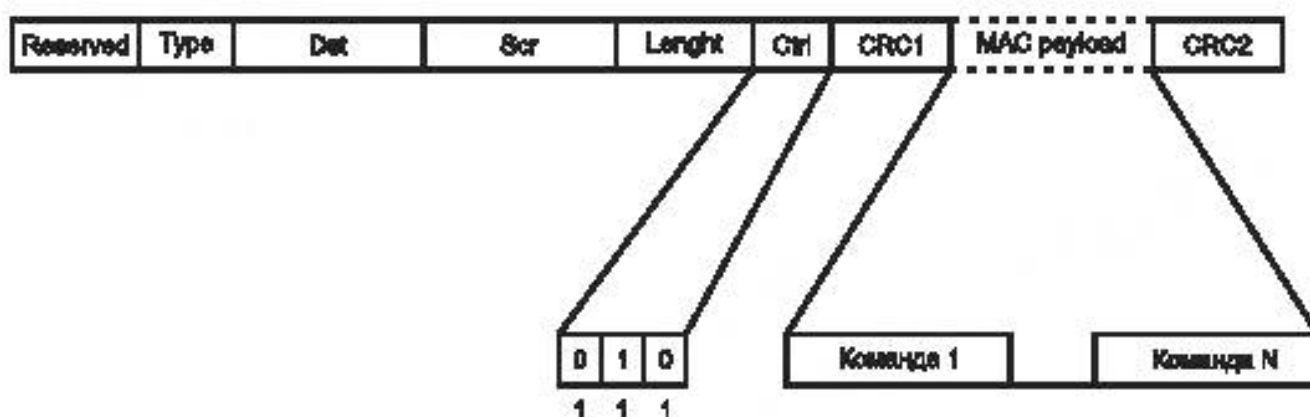
Рисунок 41 – Формат прикладного пакета команд
