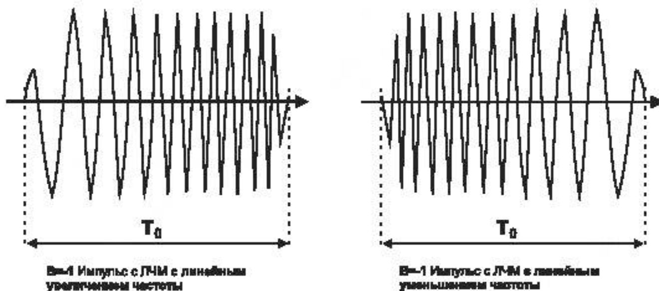
Рисунок 8 – Импульсы с ЛЧМ в полосе пропускания
