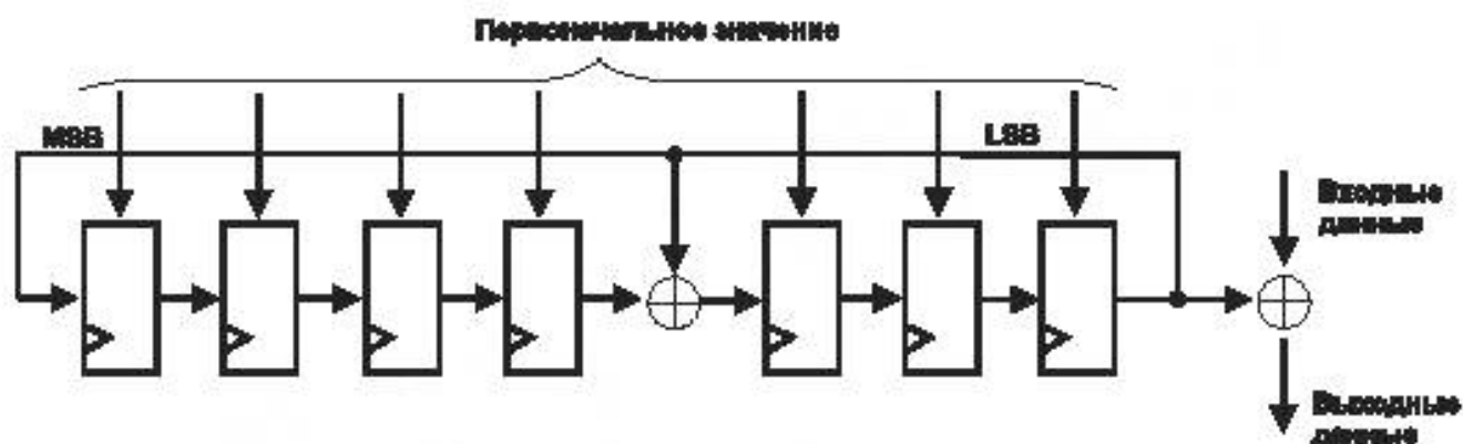
Рисунок 7 – Битовый скремблер (Bit scrambler)
