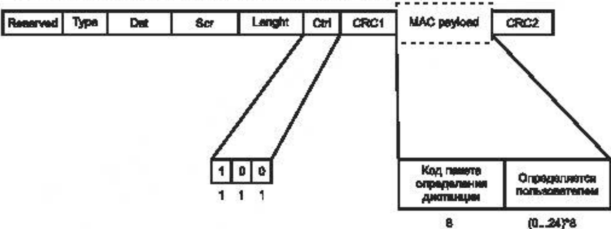
Рисунок 54 – Формат пакета измерения расстояния T4R1
