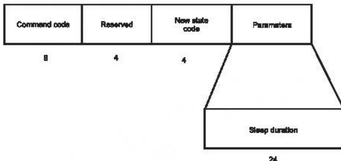
Рисунок 35 – Формат команды «Переключение в состояние «Энергосбережение» (SwitchState(Sleep))
