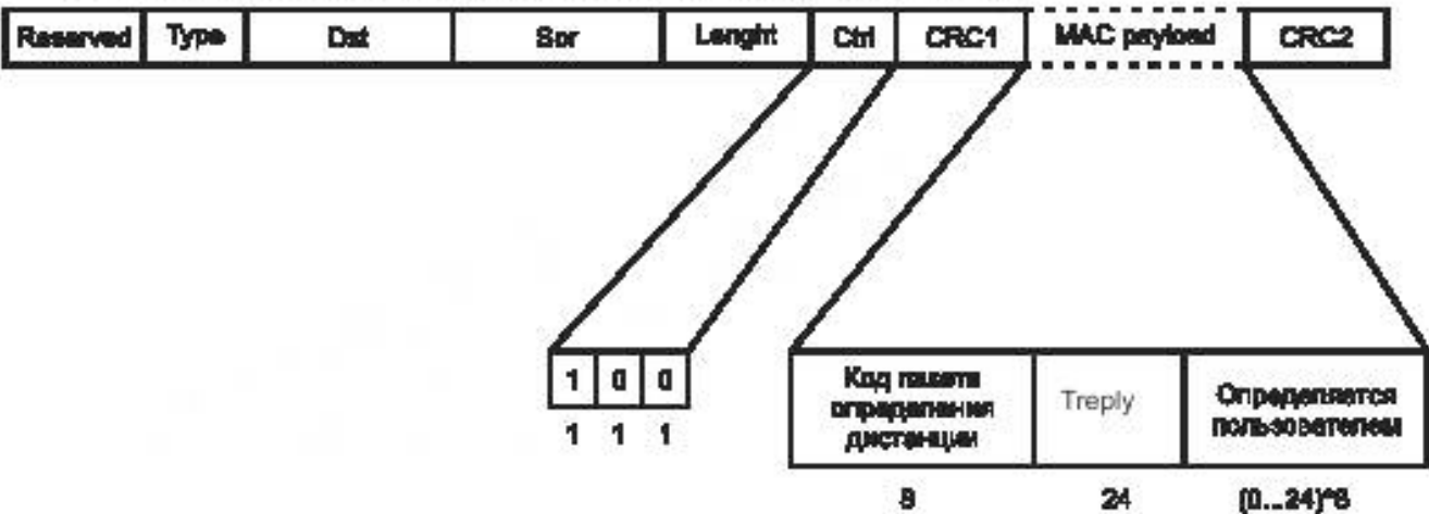
Рисунок 53 – Формат пакета измерения расстояния T3R2
