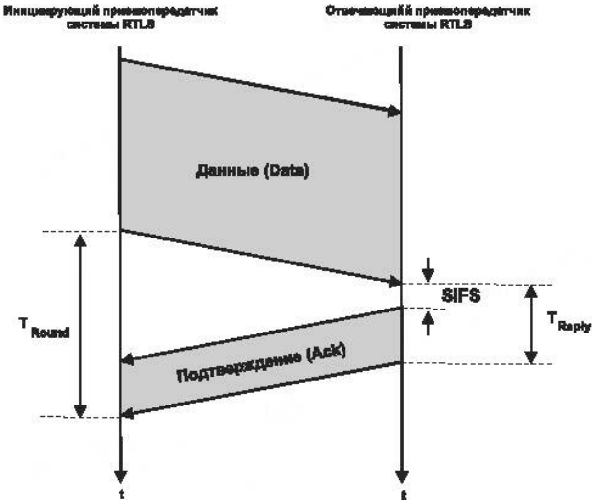
Рисунок 22 – Временные параметры подтверждения данных
