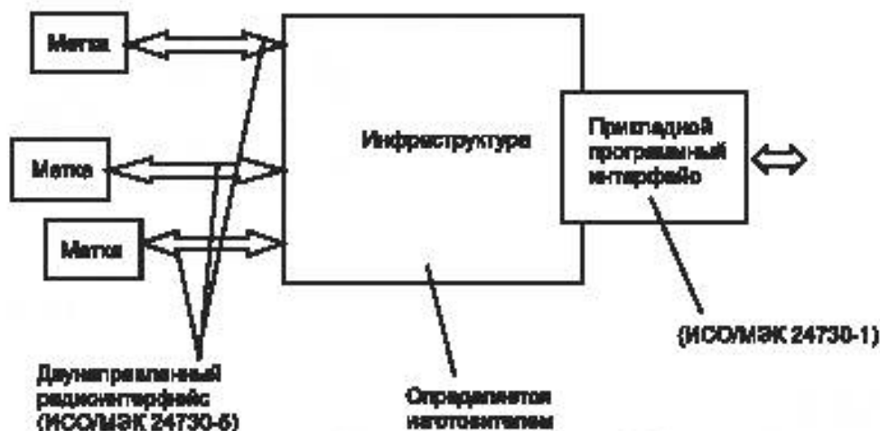
Рисунок 1 – Составные части системы RTLS
