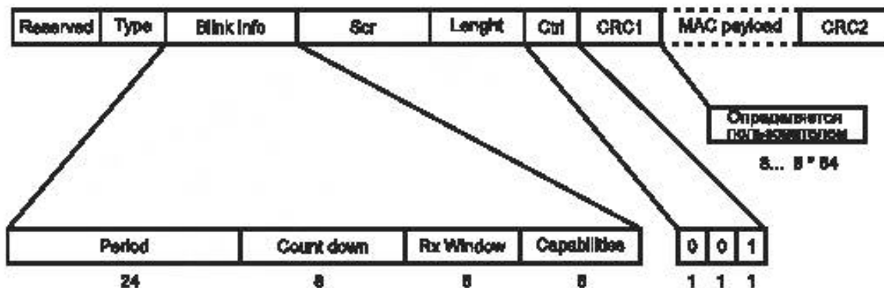
Рисунок 40 – Формат прикладного пакета передачи блинк-посылки
