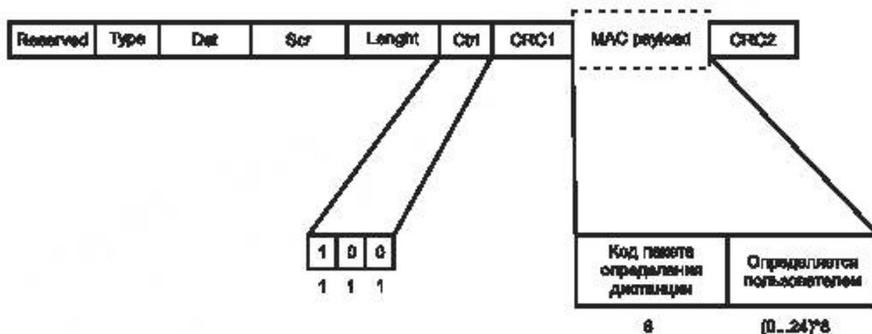
Рисунок 49 – Формат пакета измерения расстояния T2R1
