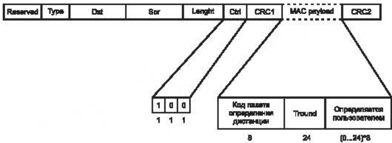
Рисунок 48 – Формат пакета измерения расстояния T1R3
