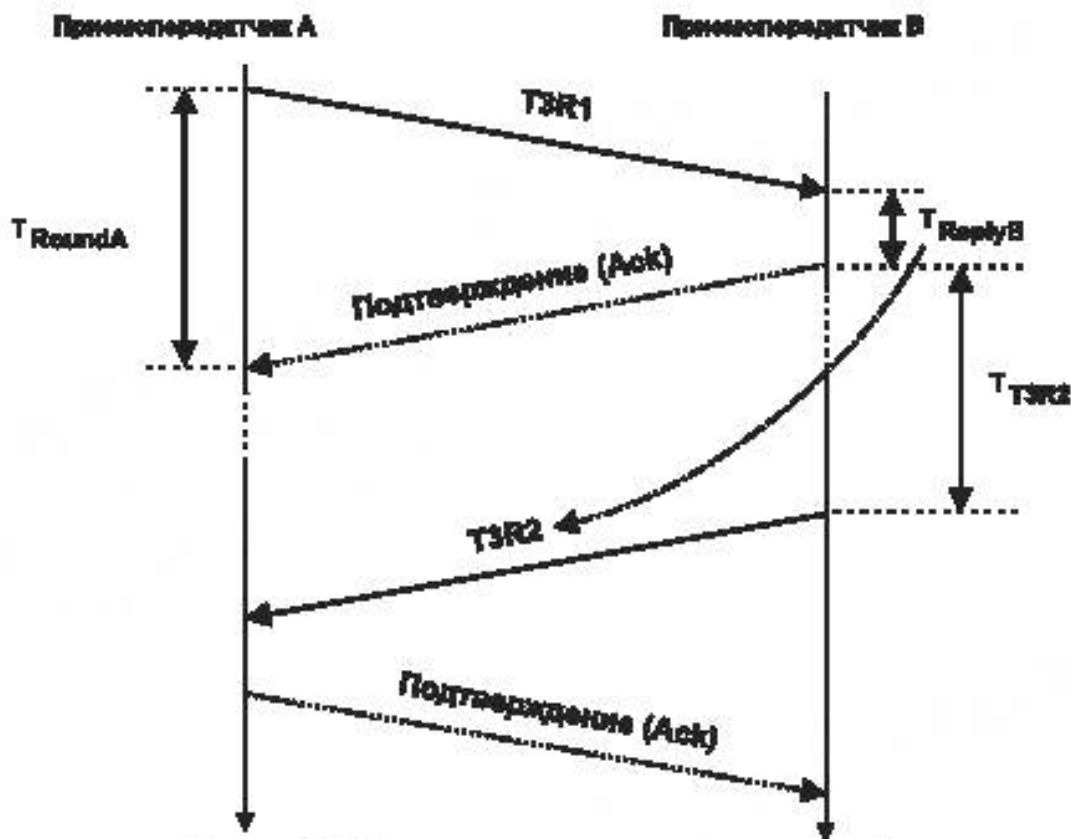
Рисунок 58 – Обмен пакетами измерения расстояния типа 3
