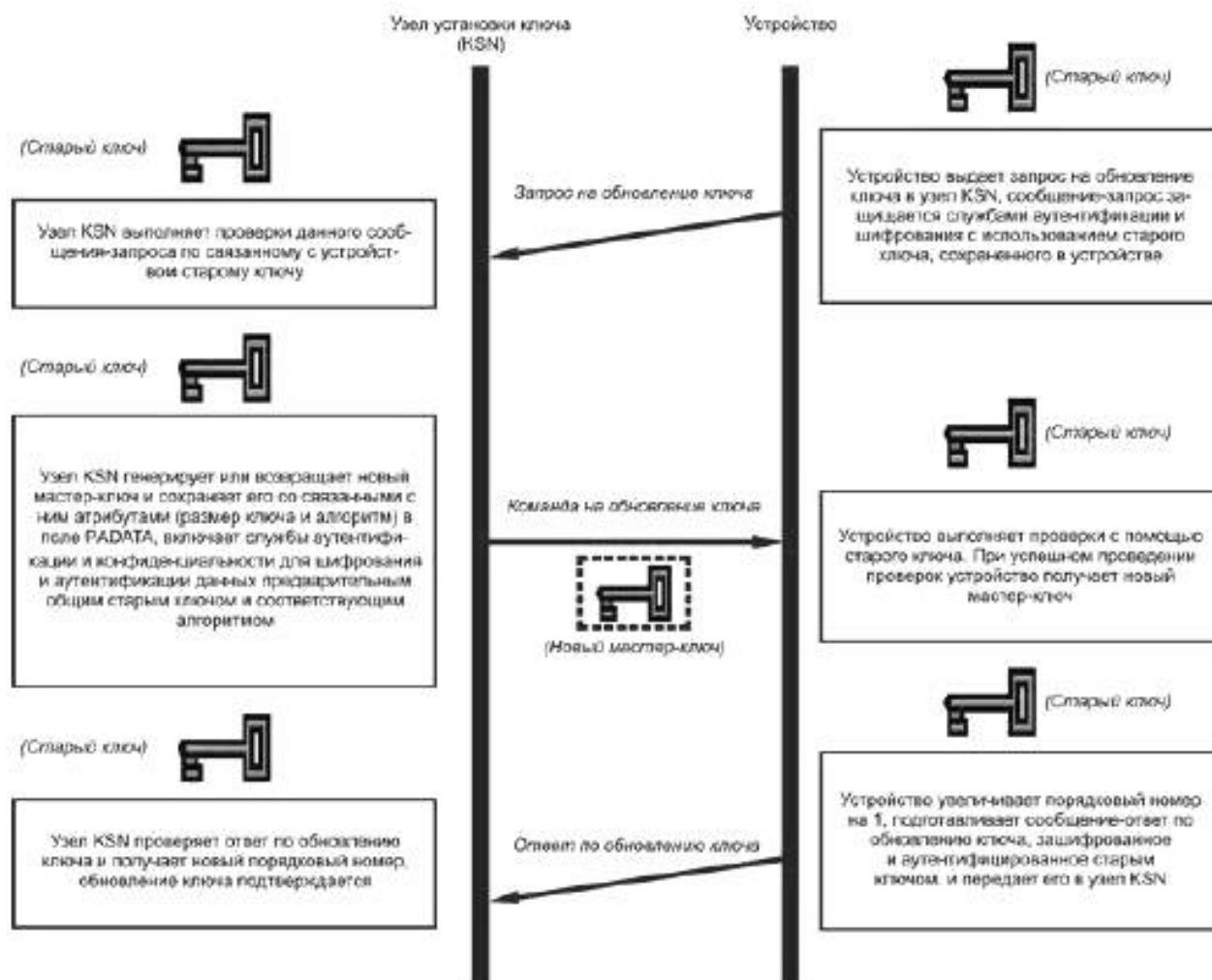
Рисунок 24 — Последовательность обновления мастер-ключа, запрашиваемого устройством
