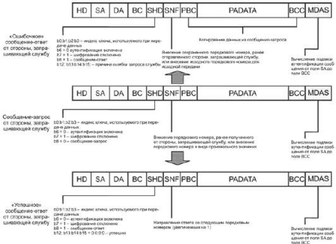
Рисунок 12 — Кадры защищенного сообщения, использующие службу удостоверяющей подписи
