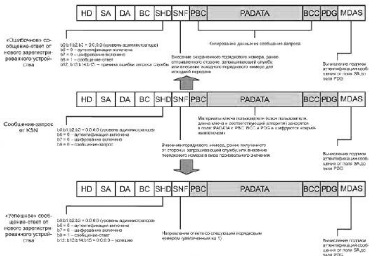
Рисунок 16 — Кадры защищенного сообщения об инициализации ключа пользователя
