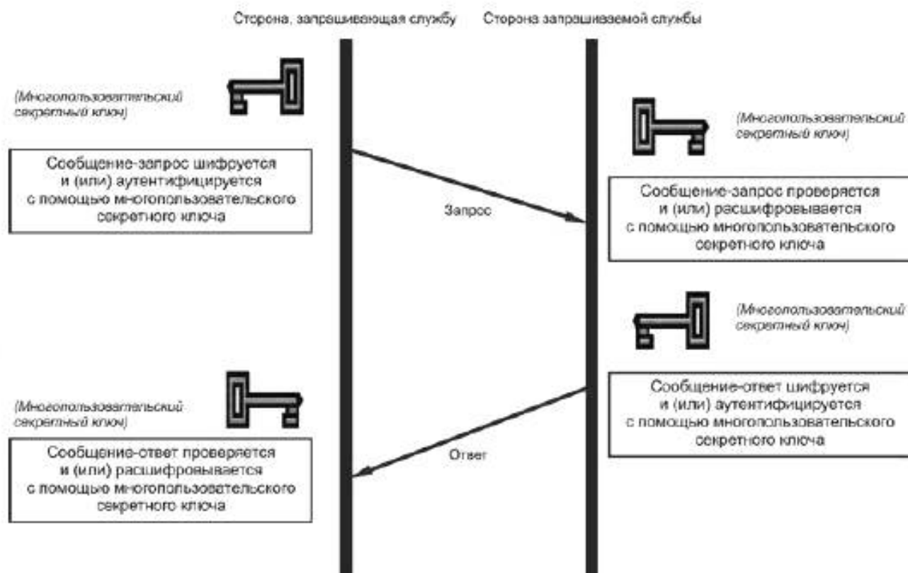
Рисунок 3 — Взаимодействие сторон на основе протокола SCPM
