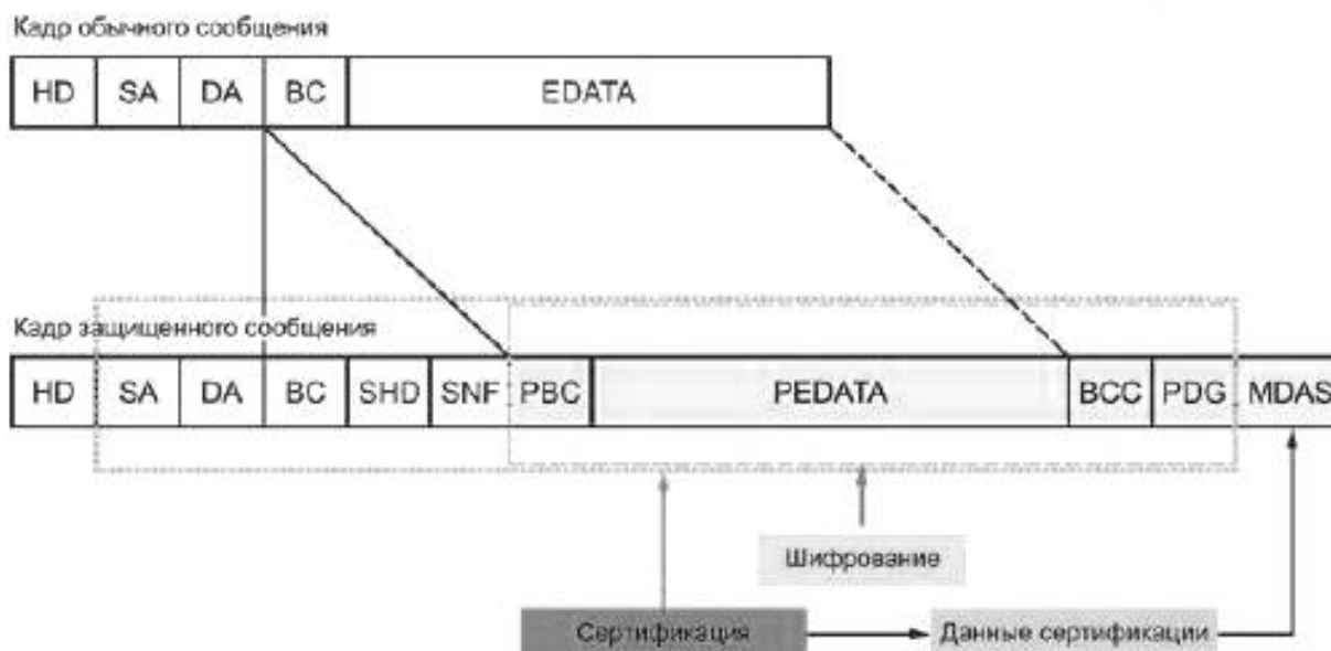
Рисунок 2 — Сравнение кадров обычного и защищенного сообщений
