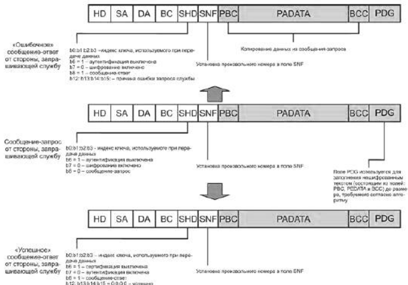
Рисунок 13 — Кадры защищенного сообщения, использующие службу шифрования
