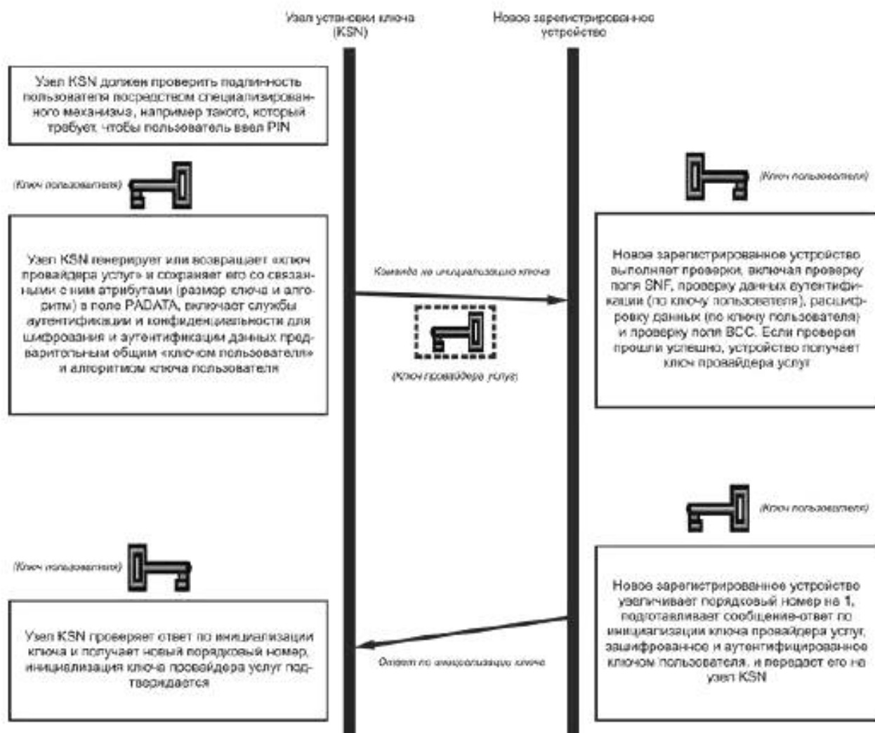
Рисунок 17 — Последовательности инициализации ключа провайдера услуг
