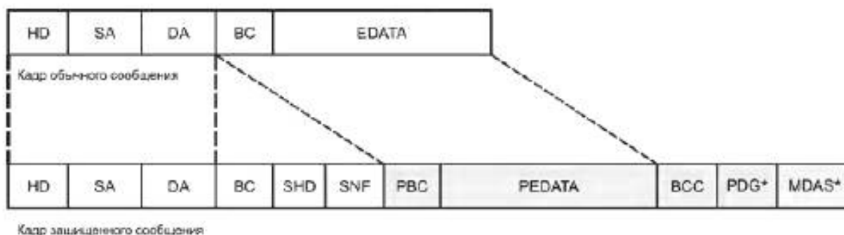
Рисунок 6 — Кадр защищенного сообщения
