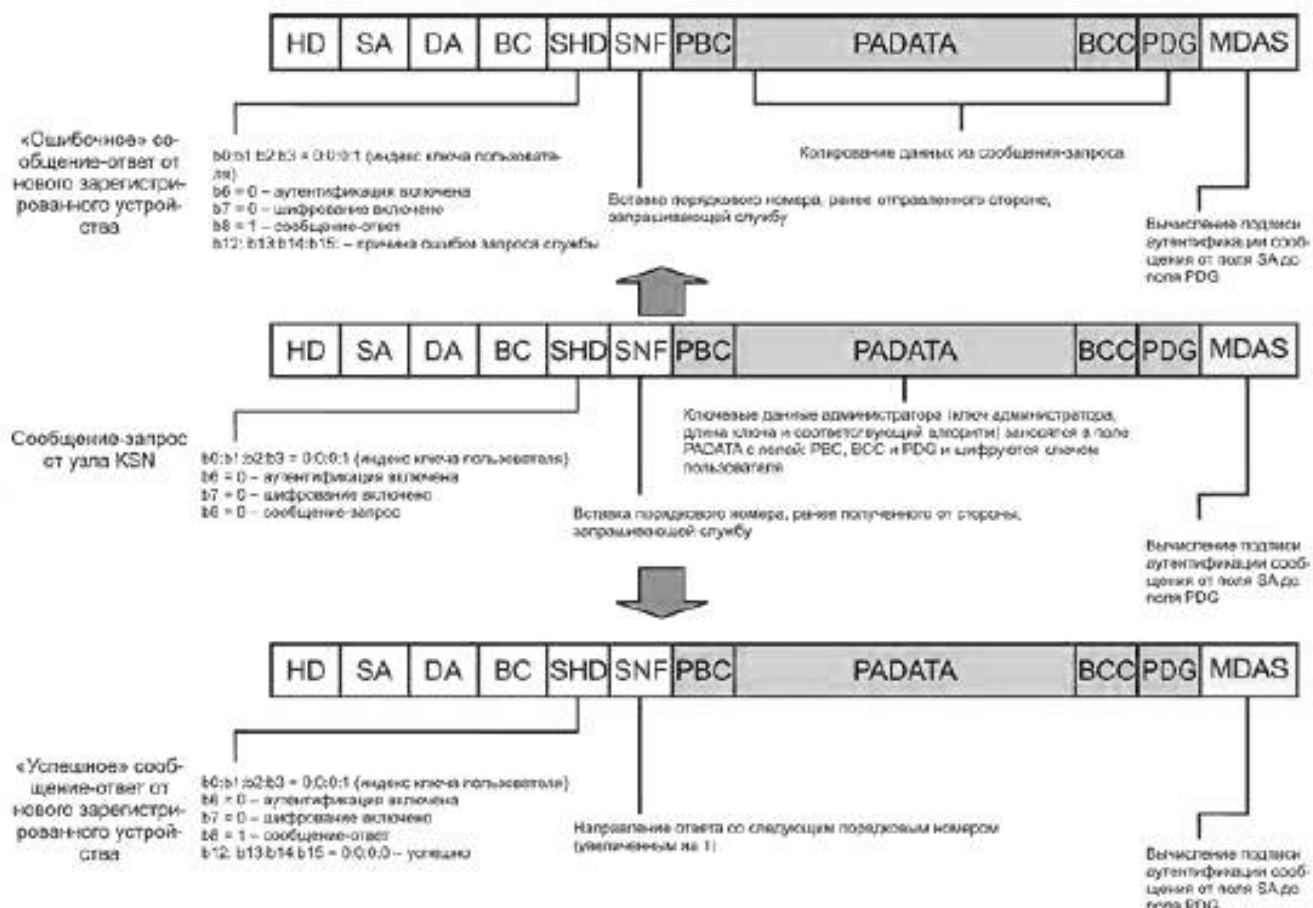
Рисунок 18 — Кадры защищенного сообщения инициализации ключа провайдера услуг
