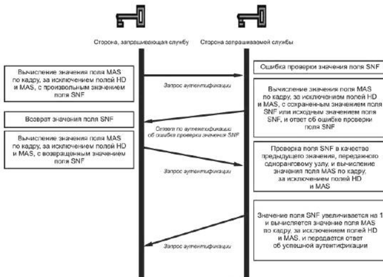
Рисунок 10 — Последовательность инициализации поля SNF
