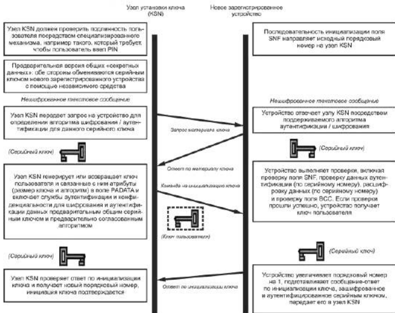
Рисунок 15 — Последовательности инициализации ключа пользователя
