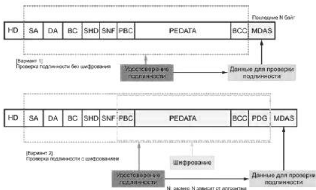
Рисунок 9 — Вычисление данных аутентификации
