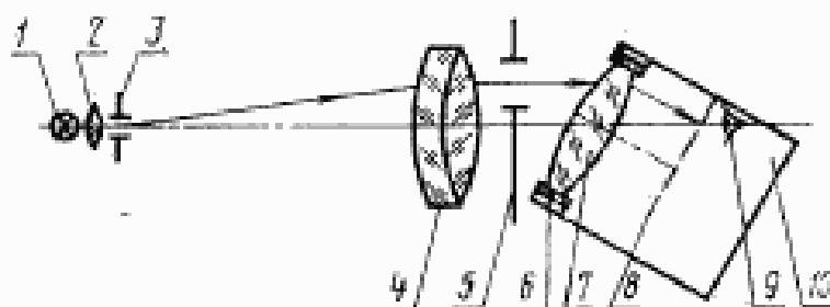
1—источник света; 2—конденсор; 3—диафрагма; 4—объектив коллиматора; 5—подвижная рамка с вертикальной нитью; 6—объективодержатель; 7—испытываемый объектив; 8—фокальная плоскость испытуемого объектива; 9—глаз наблюдателя; 10—поворотное устройство
