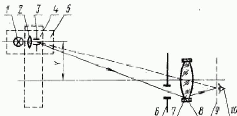
1—источник света; 2—конденсор; 3—диафрагма; 4—поперечные направляющие; 5—продольные направляющие; 6—подвижная рамка с вертикальной нитью; 7—испытываемый объектив; 8—объективодержатель; 9—плоскость изображения испытываемого объектива; 10—глаз наблюдателя
