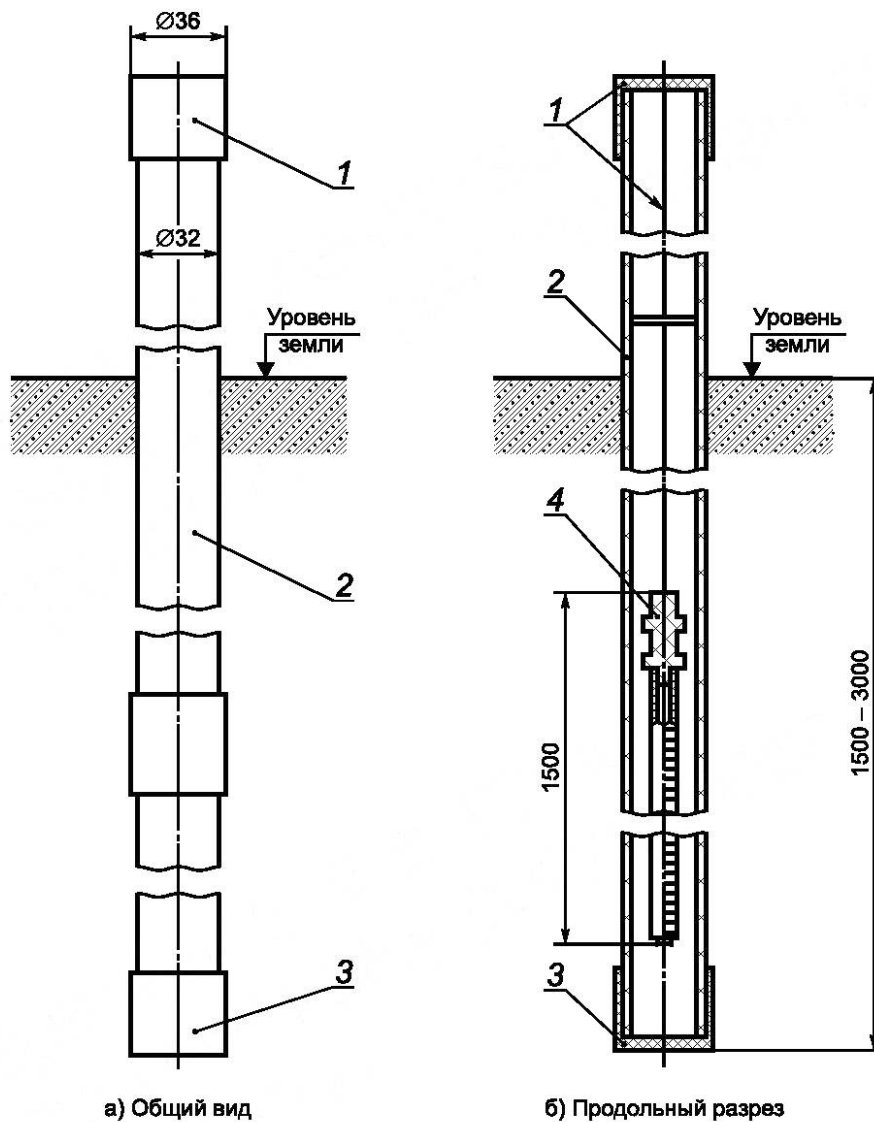
1 — верхний защитный колпачок со шнуром; 2 — защитная трубка; 3 — нижний защитный колпачок; 4 — гибкая трубка с делениями
