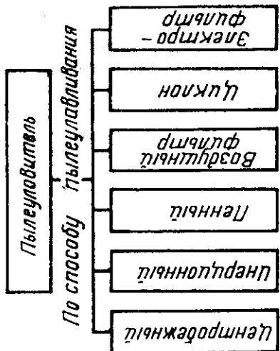
Схема 9
