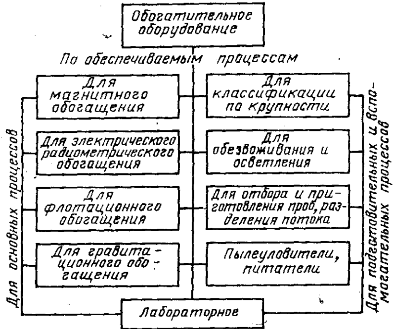
Схема 1
