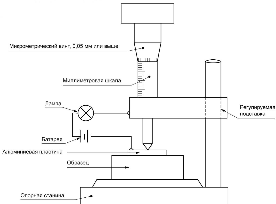
Рисунок А.1 — Пример прибора, соответствующего требованиям 4.1
