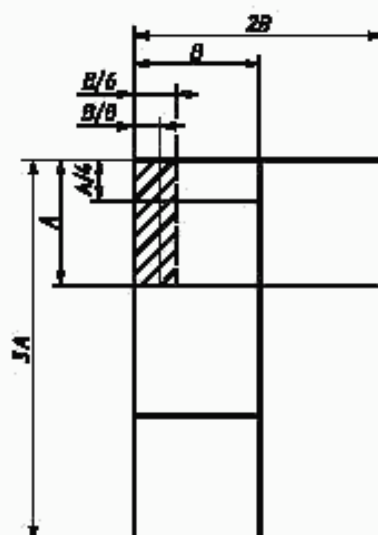
Размеры посадочных окон для панелей, устройств нестойчного типа, блочных каркасов и блоков различного назначения
