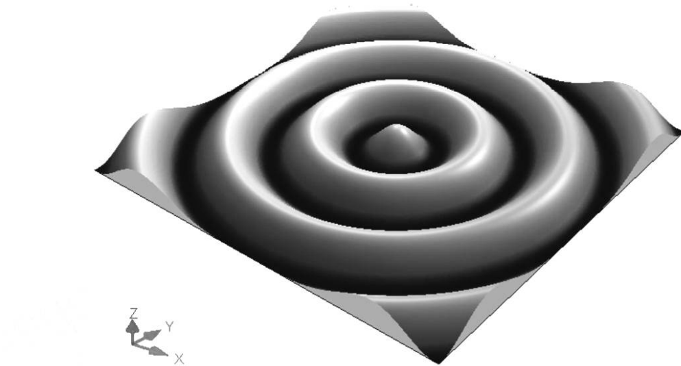
Рисунок 22 — Мера радиально-синусоидальная
