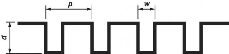
Рисунок 3 — Прямоугольный профиль
