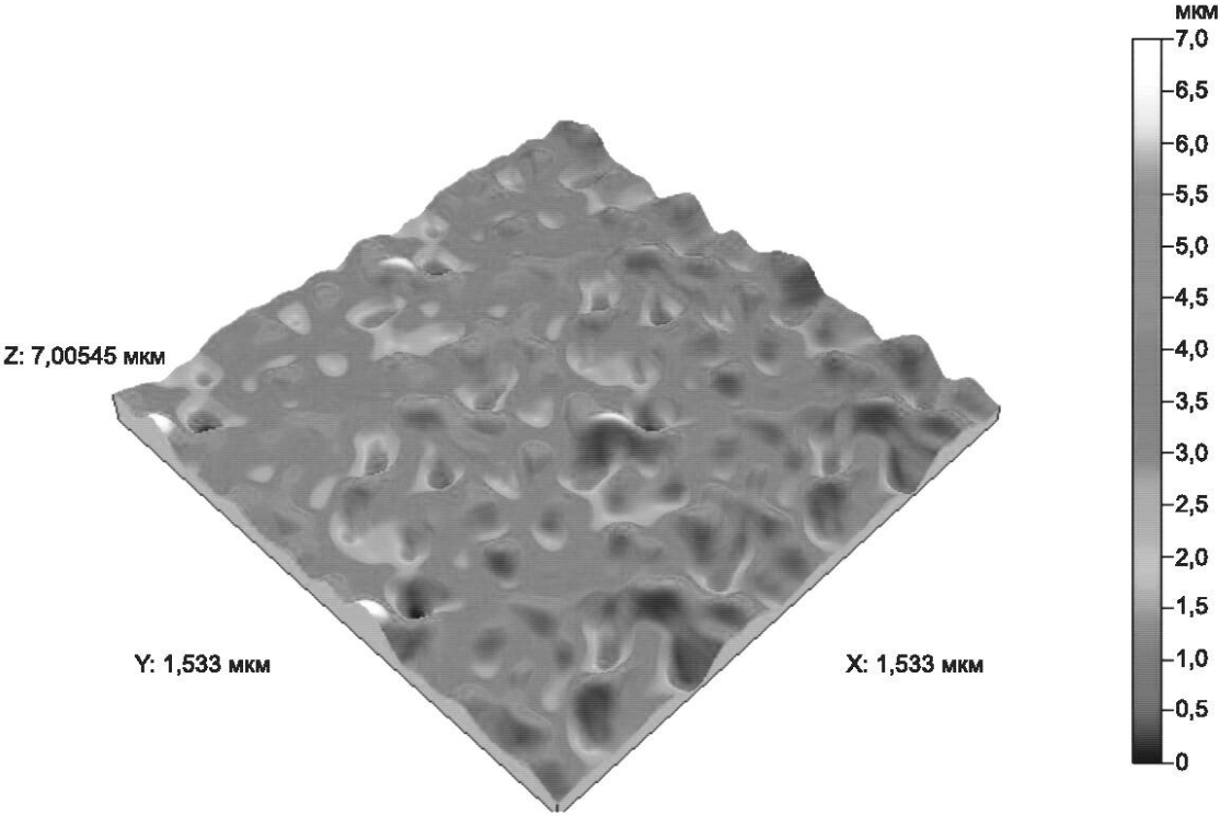
Рисунок D.2 — Результат высокочастотной механической обработки
