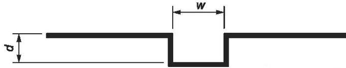
Рисунок 5 — Канавка с прямоугольной формой профиля
