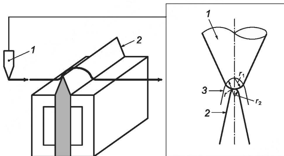
1 — щуп; 2 — лезвие бритвы; 3 — записанный профиль
