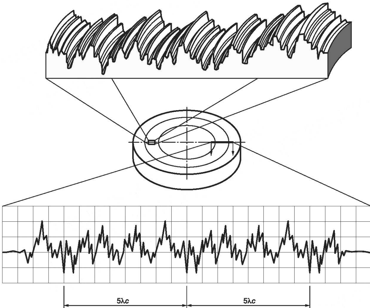
Рисунок 10 — Мера с круговым нерегулярным профилем
