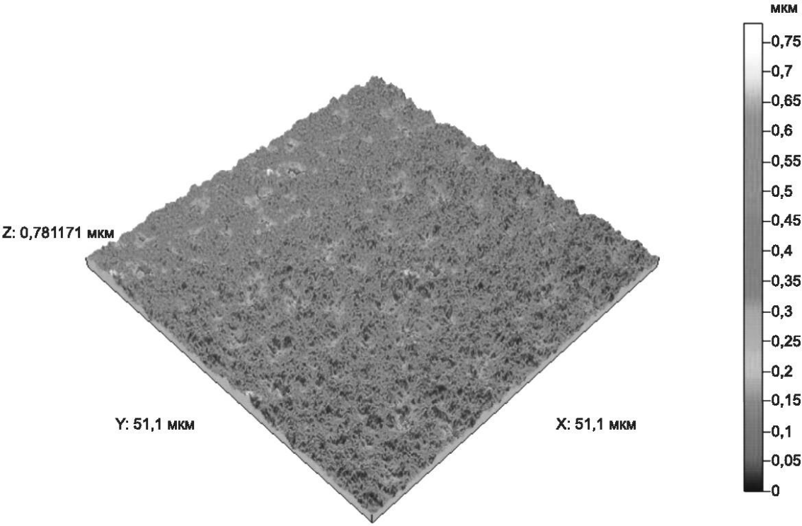
Рисунок D.1 — Результат обработки сфокусированным ионным пучком ( \beta_x = \beta_y )
