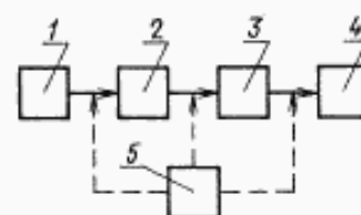
1 — исследуемый лазер; 2 — ослабитель; 3 — оптическая система; 4 — измеритель энергии; 5 — средство юстировки
