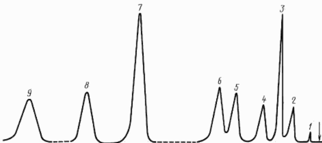
Хроматограмма искусственной смеси этиламинов
