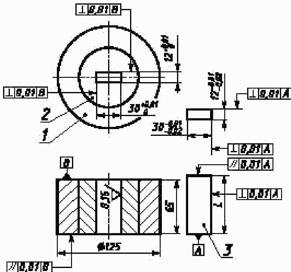
Рисунок А.1 — Пресс-форма для прессования прямоугольных образцов
