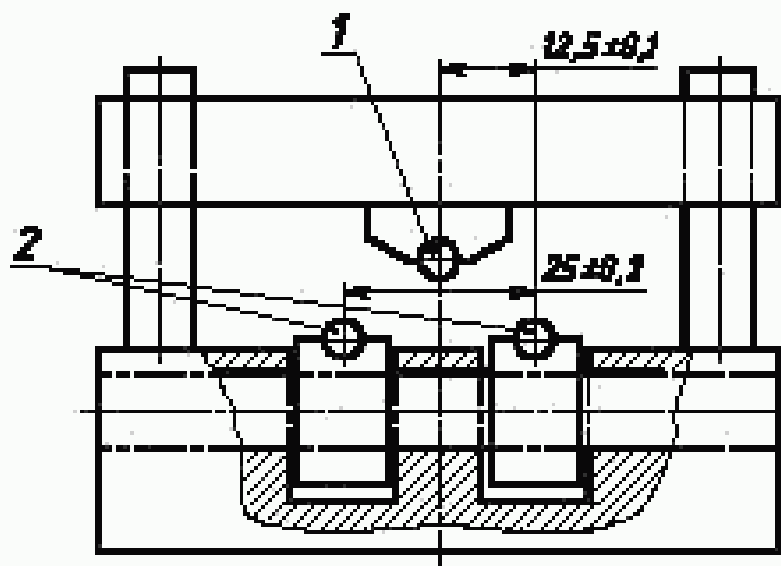
1 — нагружающий ролик; 2 — опорный ролик.
