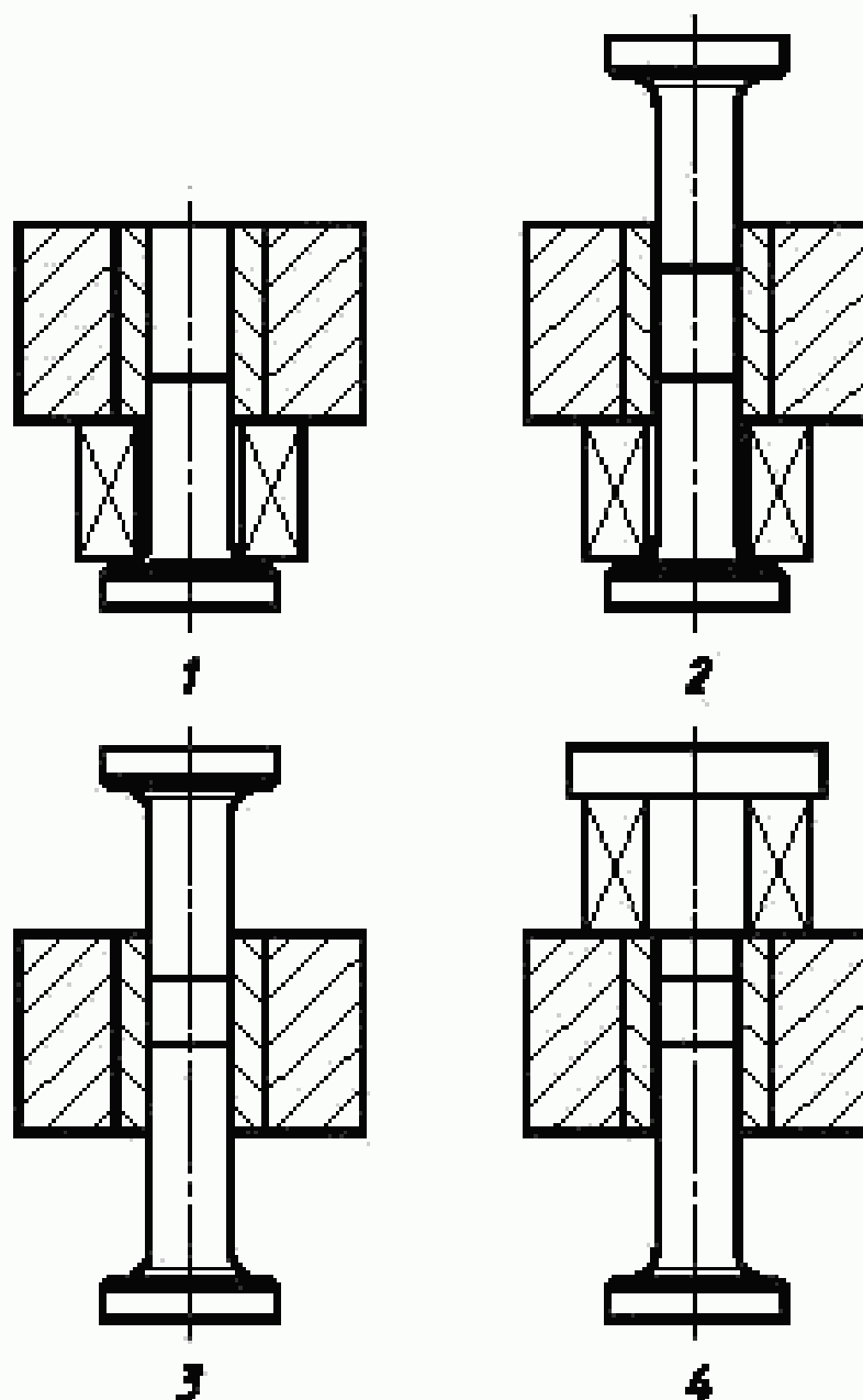
1 — загрузка; 2 — предварительное прессование; 3 — прессование; 4 — выпрессовывание
