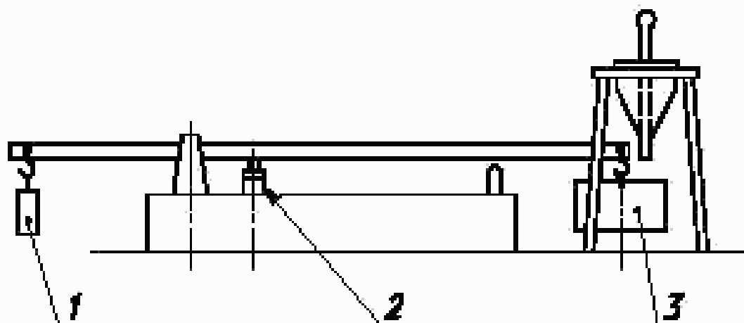
Рисунок А.3 — Устройство для нагружения
