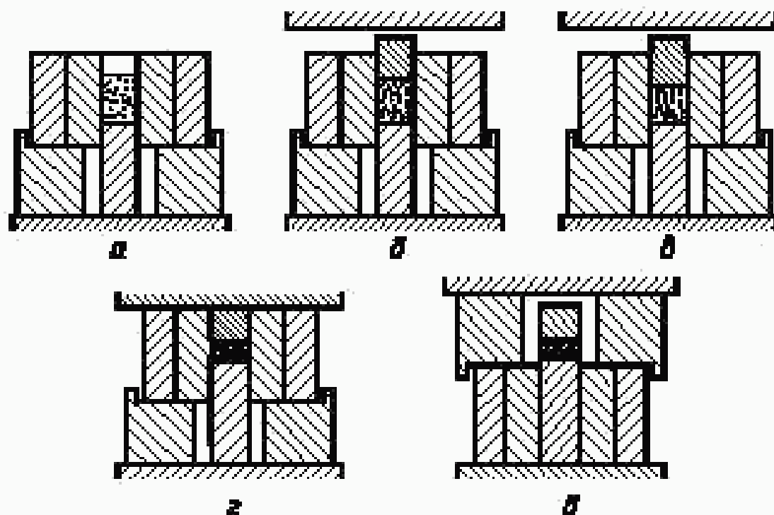
а — засыпка порошка в пресс-форму; б — установка верхнего пуансона; в — предварительное прессование; г — установка опор и окончательное прессование; д — выталкивание
