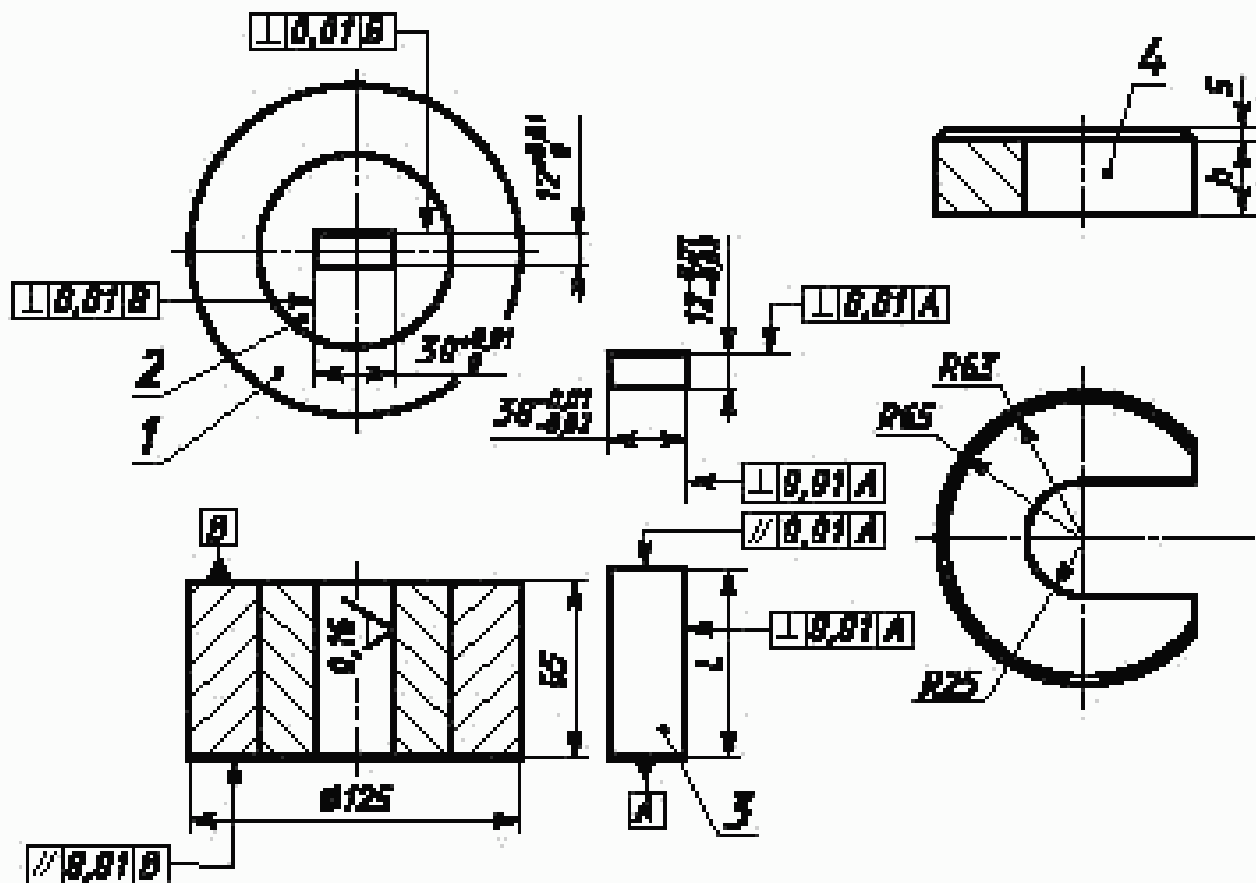
1 — обойма; 2 — матрица; 3 — пуансон; 4 — стержень
