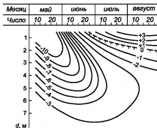
Рисунок Г.2 — Пример графика термоизоплет (термохроноизоплет) для скважины глубиной d по данным стационарных (длительных) температурных наблюдений
