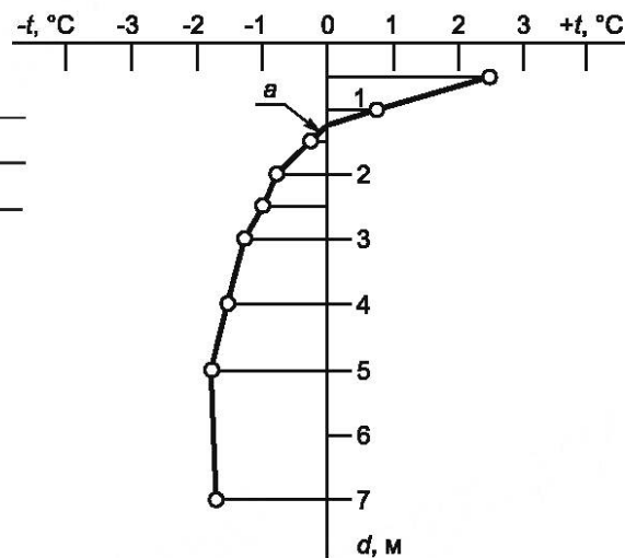
Рисунок Г.1 — Пример графика распределения температуры t , °C, грунта в скважине глубиной d для одноразовых измерений температуры
