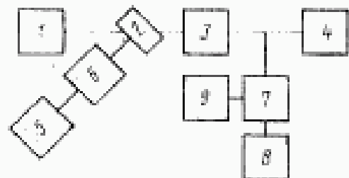
1—источник импульсов оптического излучения на основе лазера; 2—делительная пластина; 3, 4—измерительные ослабители; 4—СИ ММ с известными параметрами; 5—контрольное средство измерений; 6—камера с исследуемым фотоэлементом; 7—источник питания фотоэлемента; 8—импульсный вольтметр или осциллограф
