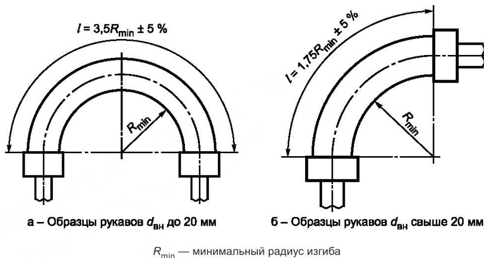
Рисунок 3 — Схема изгиба рукавов при динамических испытаниях
