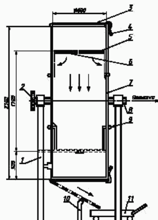
1 — система фиксирования в вертикальном положении; 2 — приводная система; 3 — сбрасывающая плита; 4 — закрепляющее устройство; 5 — фиксированная дверца; 6 — замок дверцы; 7 — кожух; 8 — оттяжка; 9 — защелка; 10 — ограничитель сыпания; 11 — контейнер
