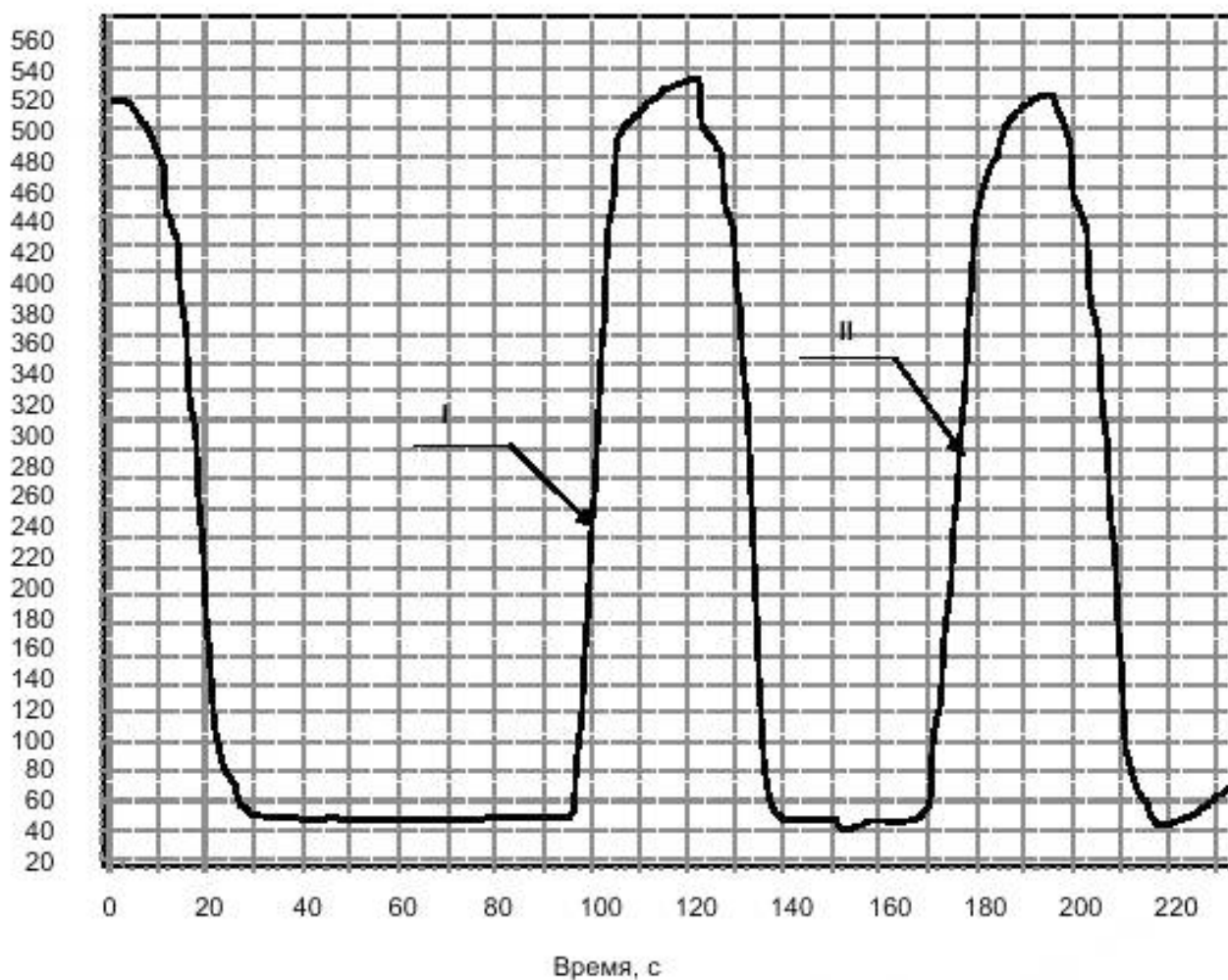
Рисунок Б.1 – Вид поляризационной кривой кулонометрического титрования диоксида серы в виноградном соке при силе тока 50 мА
