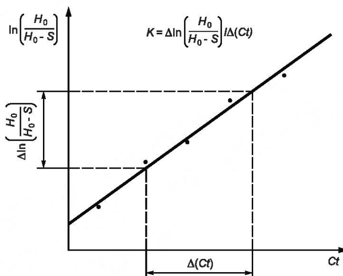
Рисунок 6 — График для определения коэффициента фильтрации глинистых грунтов
