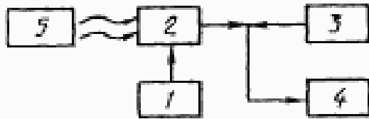
Структурная схема измерений при непрерывном воздействии
