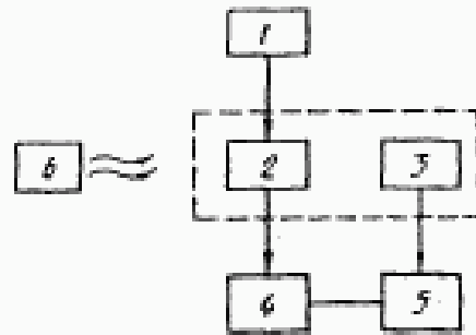
Структурная схема измерений при импульсном воздействии
