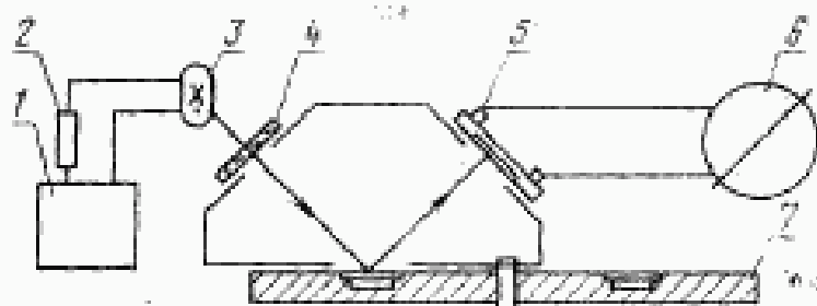
1—стабилизатор напряжения В 2-2; 2—дрозеллы; 3—бактерицидная лампа ДБ-15; 4—стеклянная пластинка, не пропускающая излучение с длиной волны 253,7 нм; 5—фотоэлемент селеновый с корректирующим фильтром ФЭС-10; 6—гальванометр типа М 195/2; 7—поворотный диск с кюветами для люминофора
