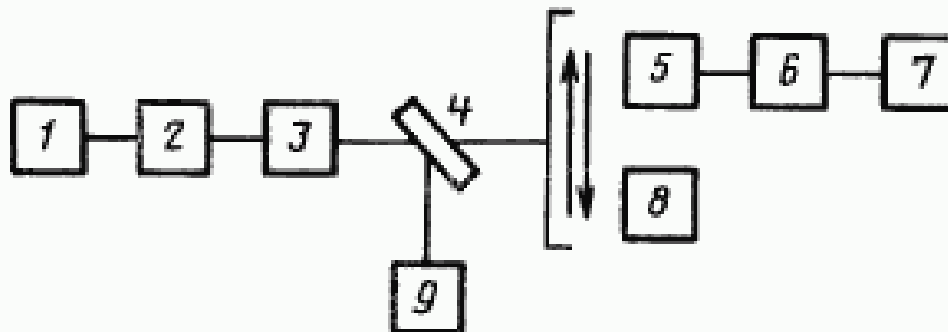
1 — лазер; 2 — модулятор; 3 — ослабитель; 4 — делительная пластинка; 5 — первичный измерительный преобразователь исследуемого средства измерений; 6 — селективный усилитель; 7 — система регистрации; 8, 9 — контрольные средства измерений
