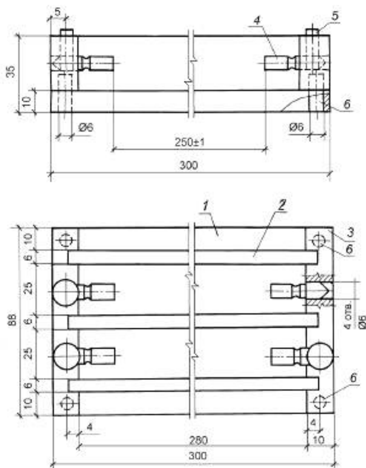
1 — доньшко формы; 2 — боковая стенка формы; 3 — торцевая стенка формы; 4 — вкладыш из нержавеющей стали; 5 — винт М5х25; 6 — штифт
