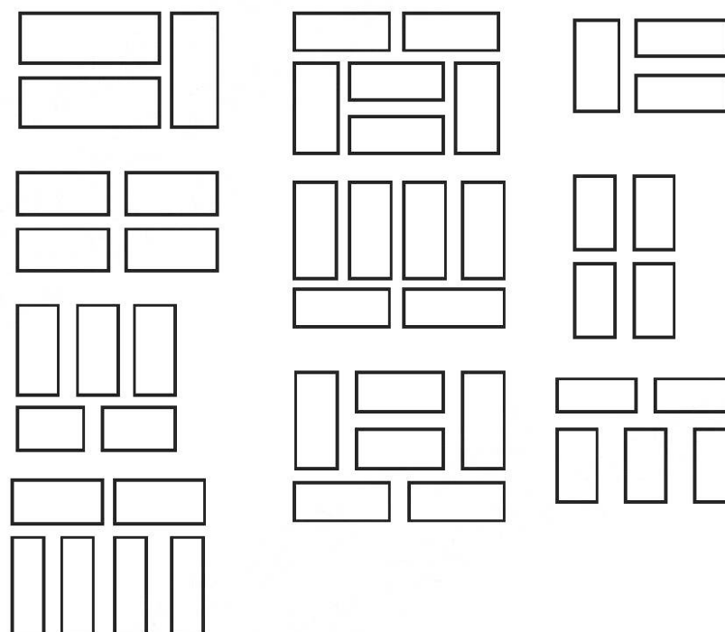
Рисунок А.1 — Рядовая укладка
