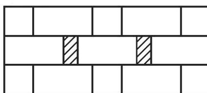
Рисунок А.2 — Укладка с образованием пустот в центре пакета
