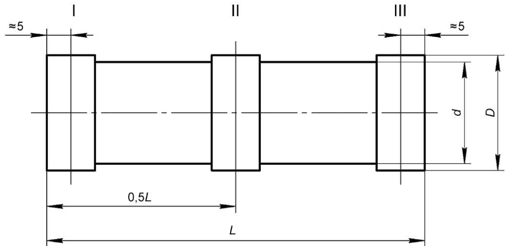
Рисунок 1 — Форма образца-изделия
