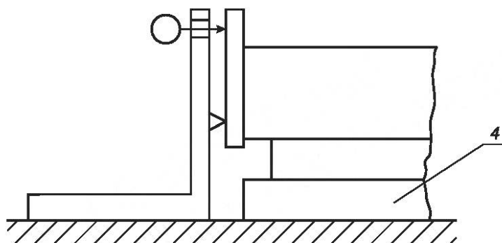
Рисунок 4 — Схема проверки с помощью специального проверочного приспособления, устанавливаемого на поверочной плите (метод 1)
