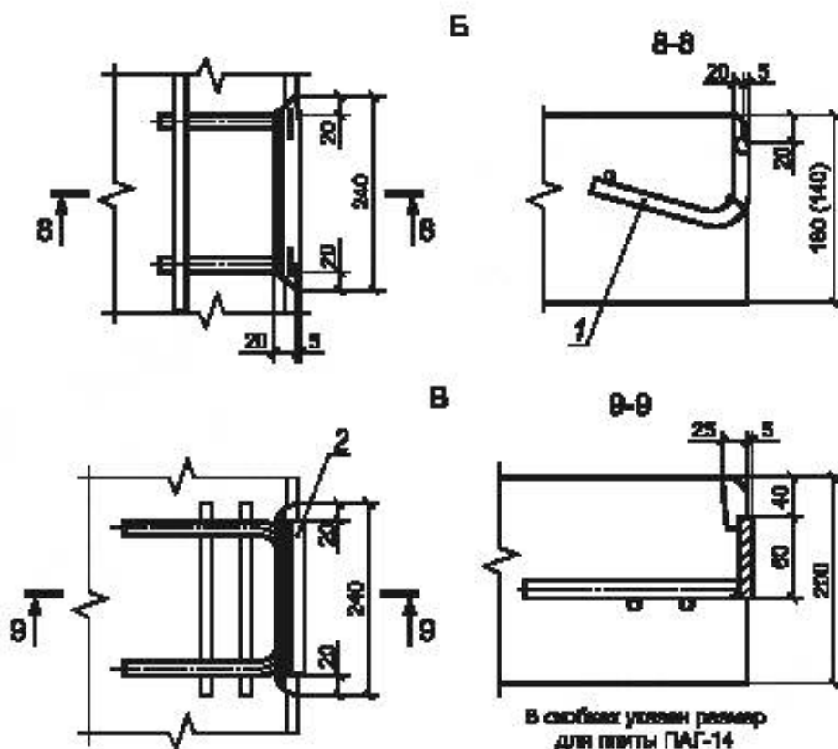
1 — стыковое изделие М2 (М2в) или М4 (М4в); 2 — стыковое изделие М4а; М2в и М4в — маркировка з/д для ПАГ-14А800-1 и ПАГ-18А800-1
