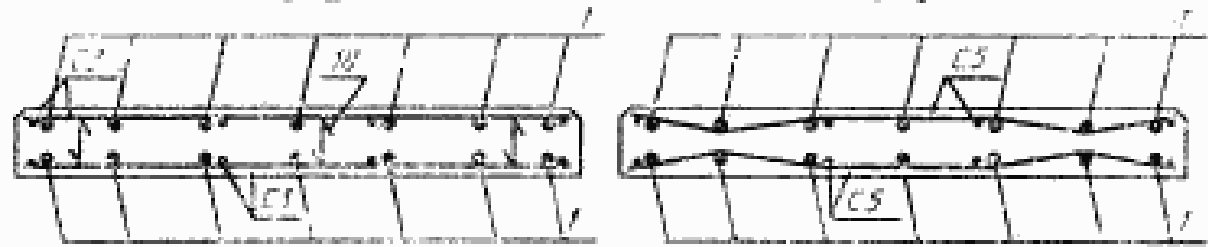
1 — напрягаемая арматура; 2 — крепление сеток C3
