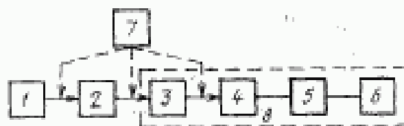
1—лазер; 2—ослабитель; 3—оптическая система; 4—матричный преобразователь; 5—коммутирующее устройство; 6—измерительный прибор; 7—средство юстировки; 8—средство измерения ОРПЭ (М)
