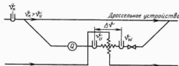
Дроссельное устройство
