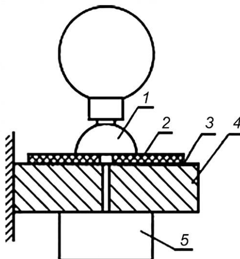
1 — испытуемый электрод; 2 — уплотнительный лист (например, из мягкой резины, ориентировочные размеры: 3 × 50 × 50 мм); 3 — слой клея; 4 — основание; 5 — вакуумметр
