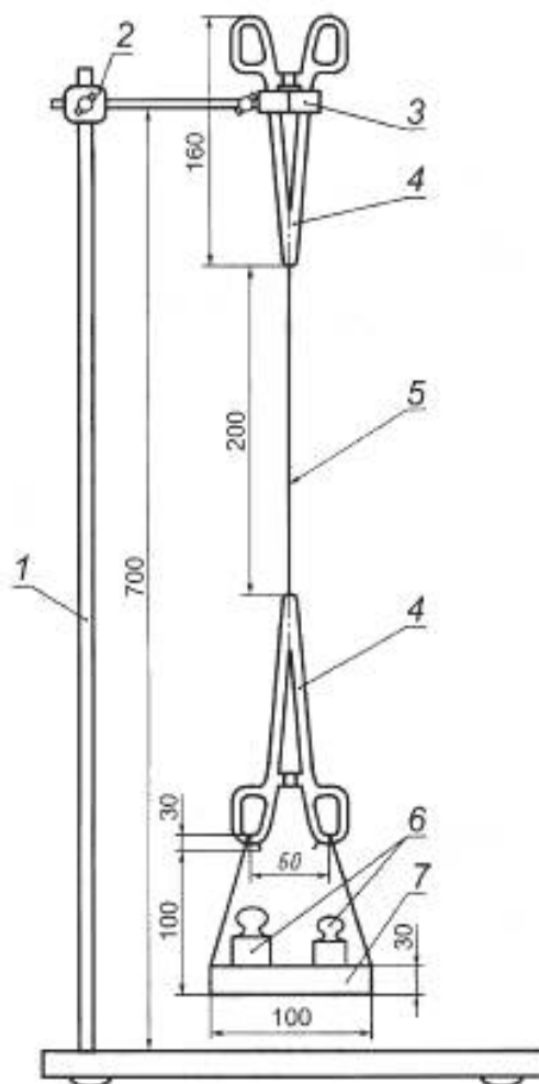
1 — штатив; 2 — муфта; 3 — зажим; 4 — зажим с кремальерой; 5 — лист филлоспадикса или зостеры; 6 — груз; 7 — квадратная коробка с проволоочными крючками (для груза)
