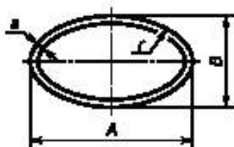
A — большая ось; B — малая ось; r — радиус закругления; S — толщина стенки
