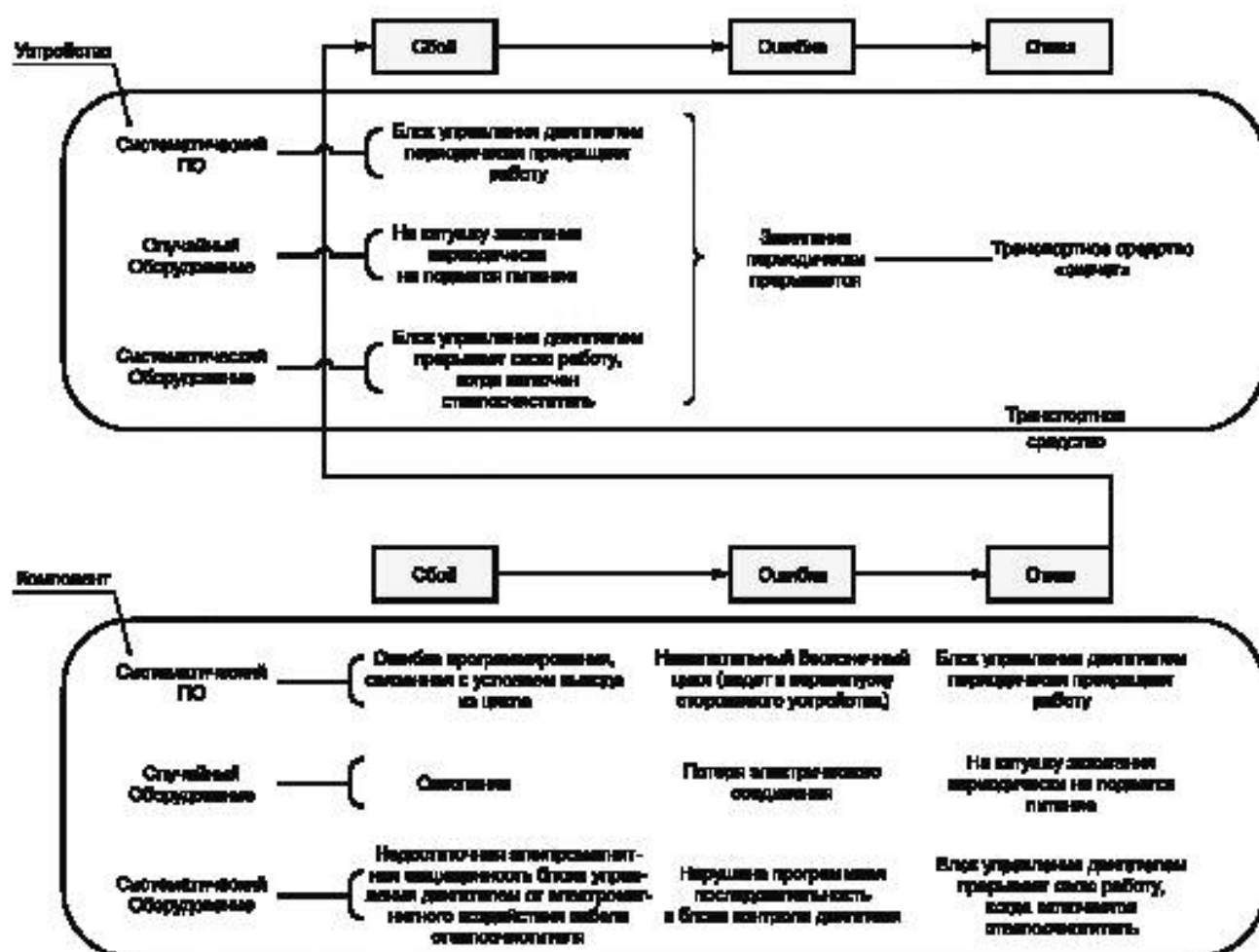
Рисунок 5 — Пример сбоев, приводящих к отказам
