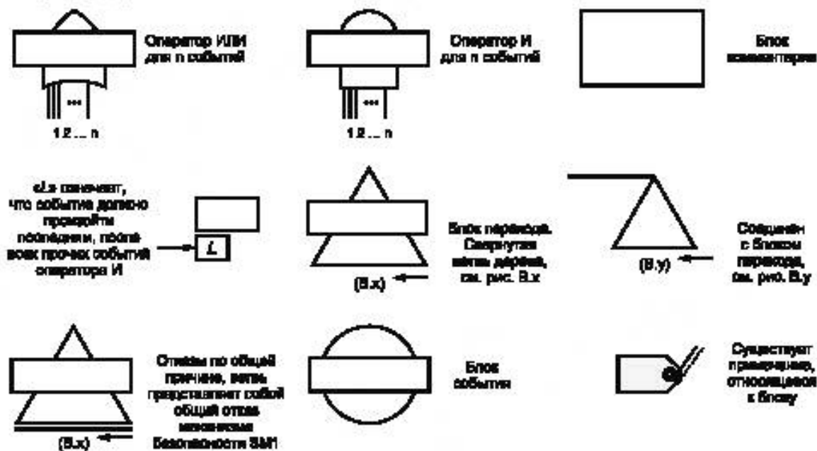
Рисунок В.5 — Краткое описание символов FTA
