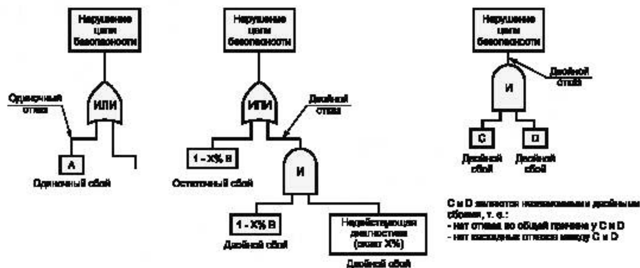
Рисунок В.4 — Примеры FTA для одиночного, остаточного и двойного сбоя
