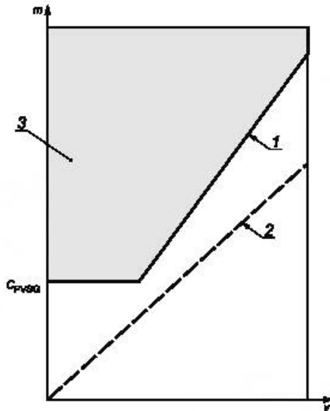
1 — связанная с безопасностью нижняя граница \mu_{\text{SafeRelAmin}} датчика A_Master; 2 — возвращаемое значение идеального датчика с нулевым допуском (как эталон); 3 — сбой с возможным нарушением цепи безопасности
