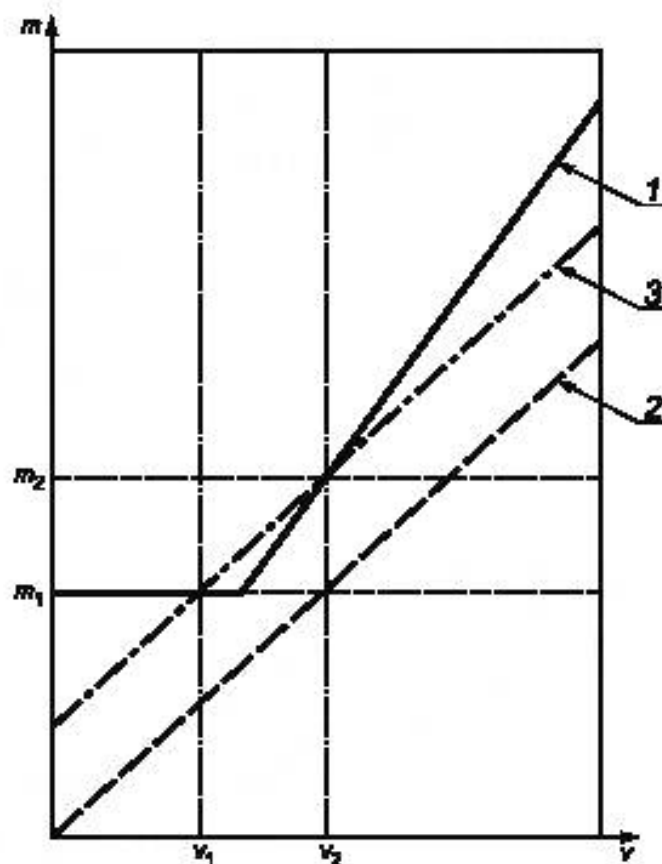
1 — связанная с безопасностью нижняя граница \mu_{SafeRel, A, min} датчика A\_Master ; 2 — возвращаемое значение идеального датчика с нулевым допуском (как эталон); 3 — наихудший случай порога обнаружения \mu_{A, Master, wc} .
