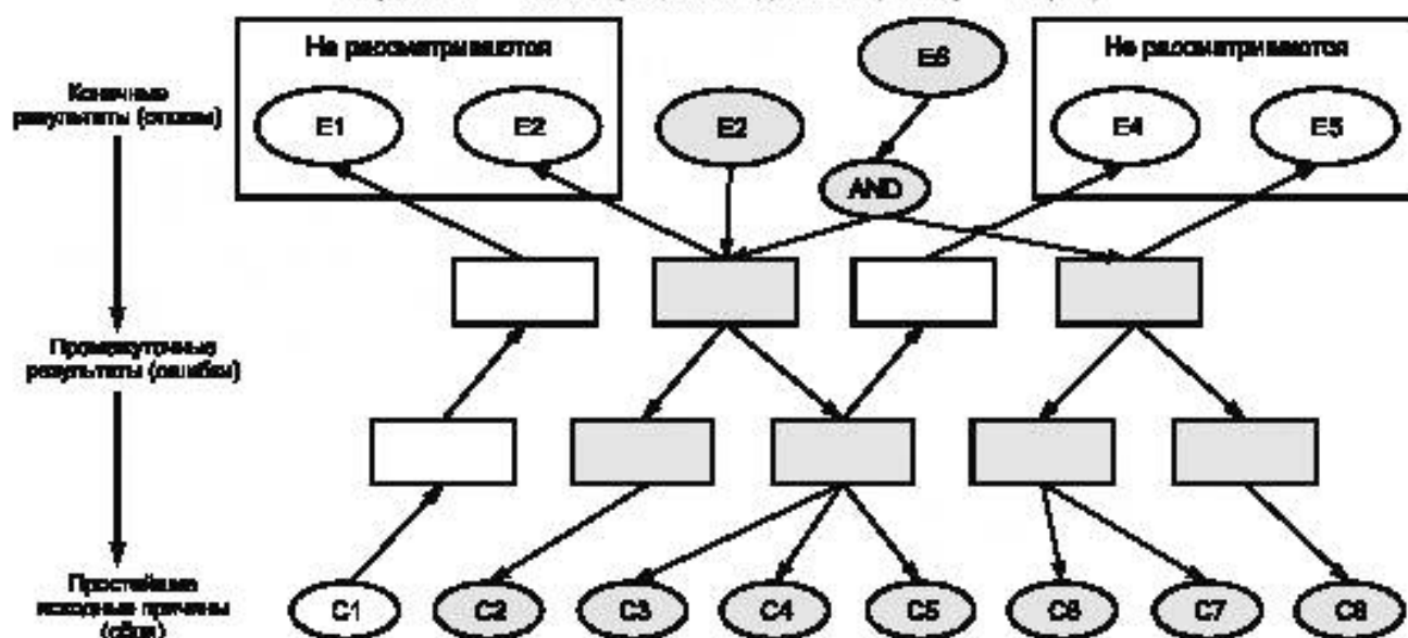
Рисунок В.2 — Иллюстрация метода FTA («сверху—вниз»)
