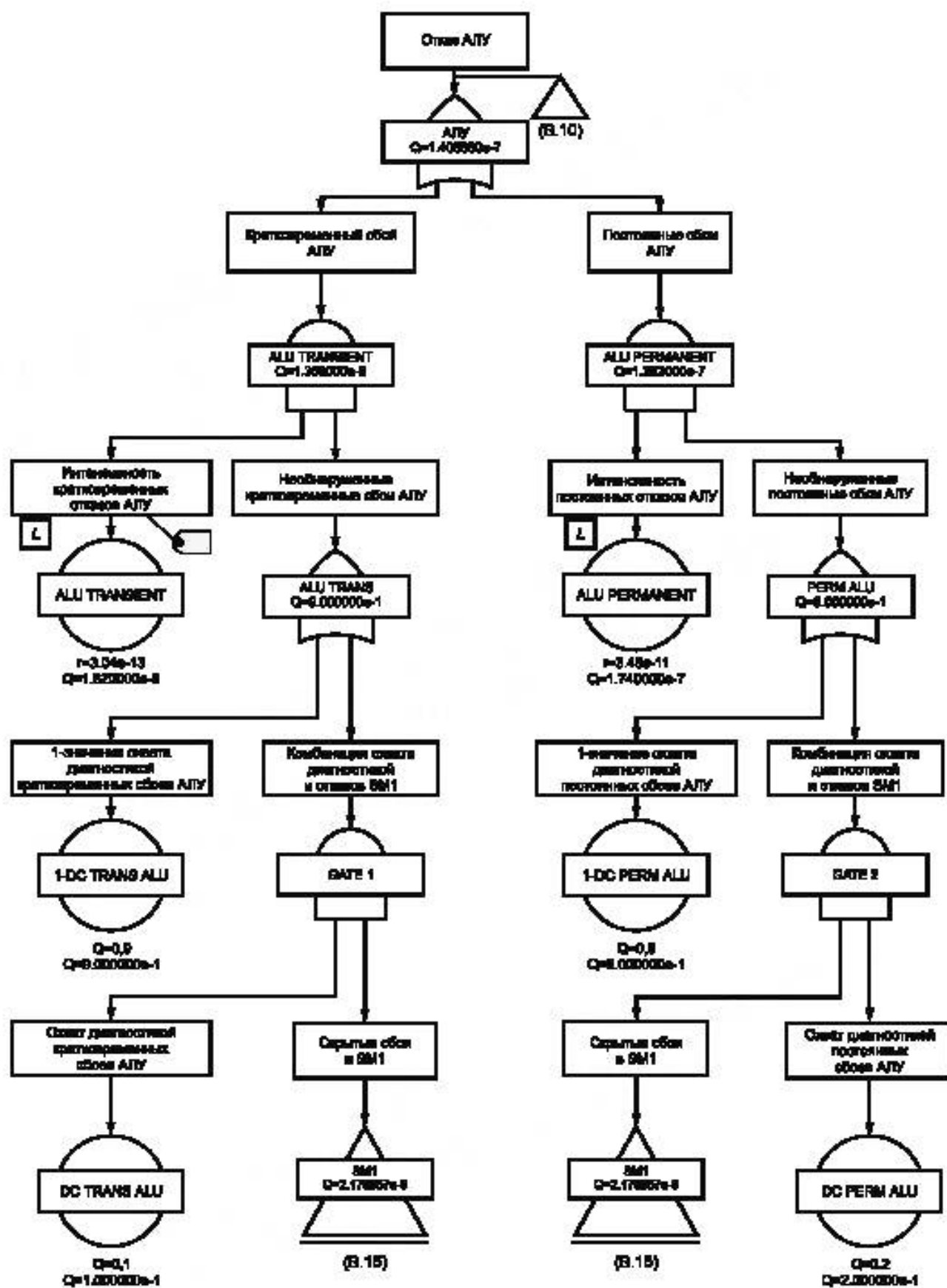
Рисунок В.11 — Ветвь дерева неисправностей, представляющая АЛУ
