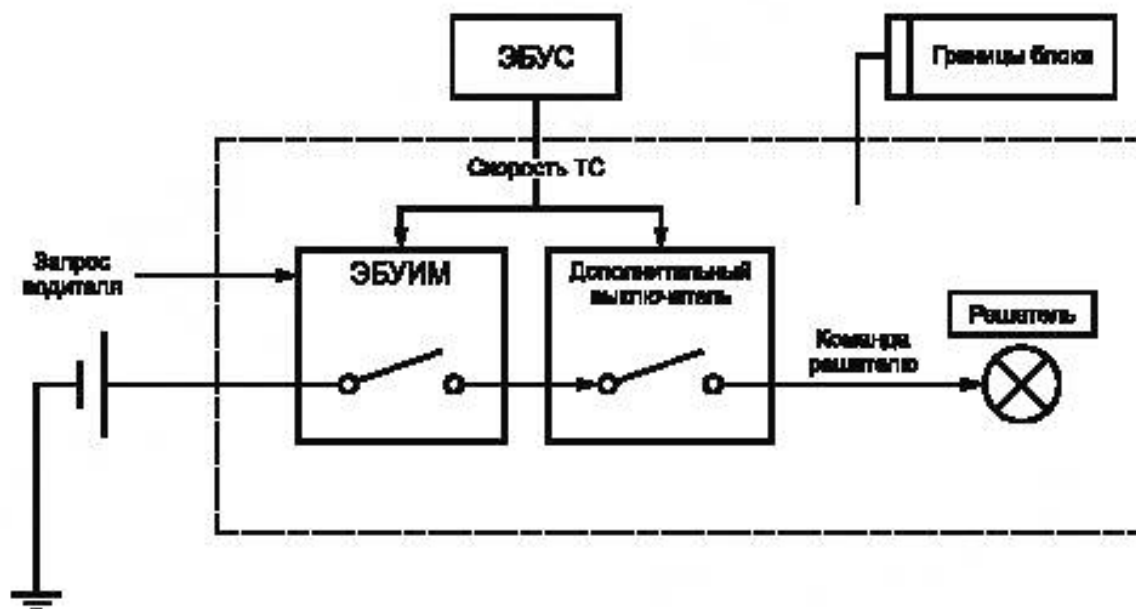
Рисунок 23 — Вторая итерация проекта устройства
