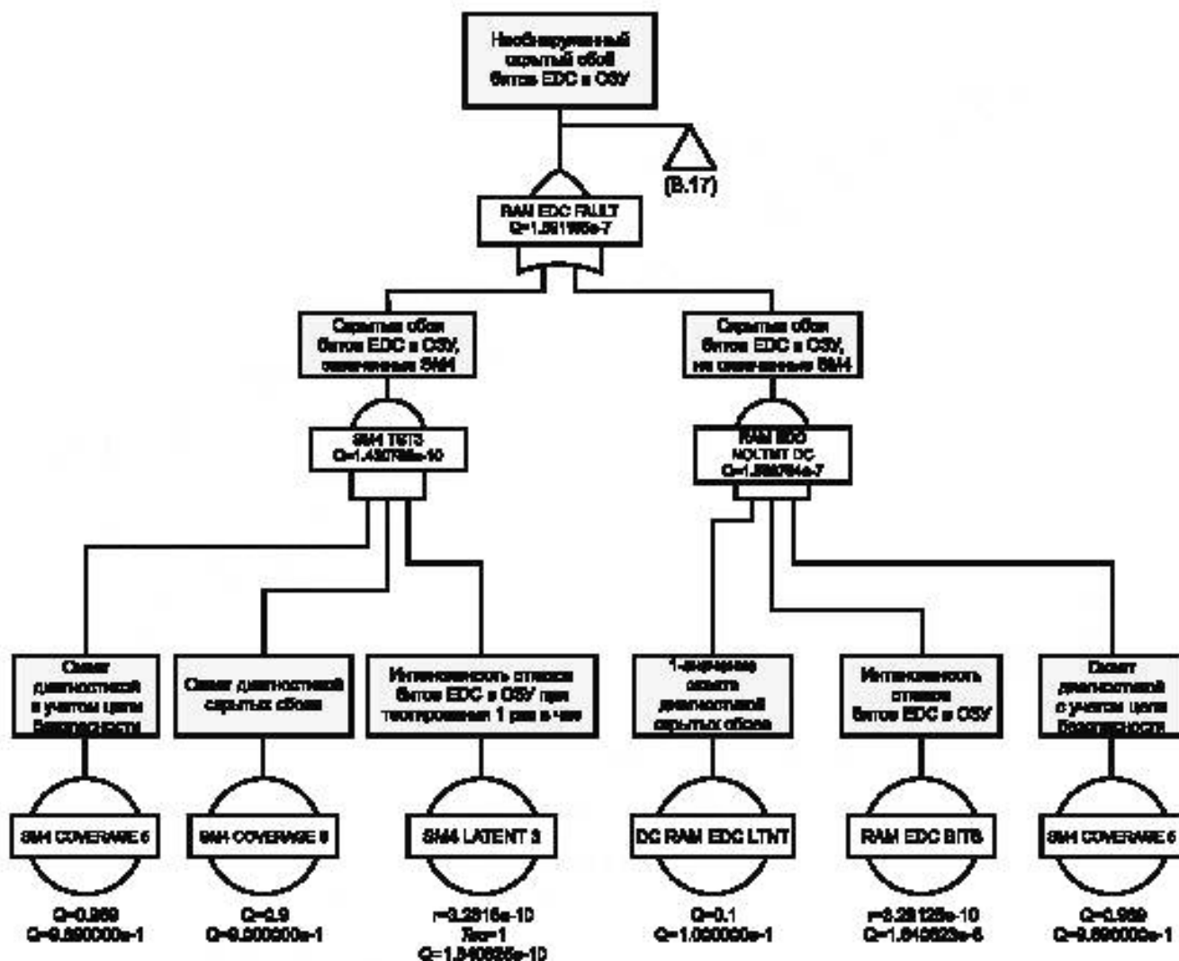
Рисунок В.19 — Ветвь дерева неисправностей, представляющая скрытые сбои битов EDC в OSU
