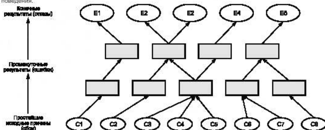
Рисунок В.1 — Иллюстрация метода FMEA («снизу — вверх»)
