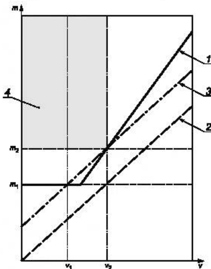
1 — связанная с безопасностью нижняя граница P_{SaRelA,min} датчика A\_Master ; 2 — возвращаемое значение идеального датчика с нулевым допуском (как эталон); 3 — наихудший случай порога обнаружения \mu_{A\_Master,wc} ; 4 — двойные обнаруживаемые сбои
