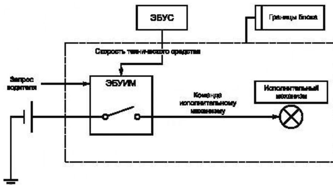
Рисунок 22 — Границы устройства
