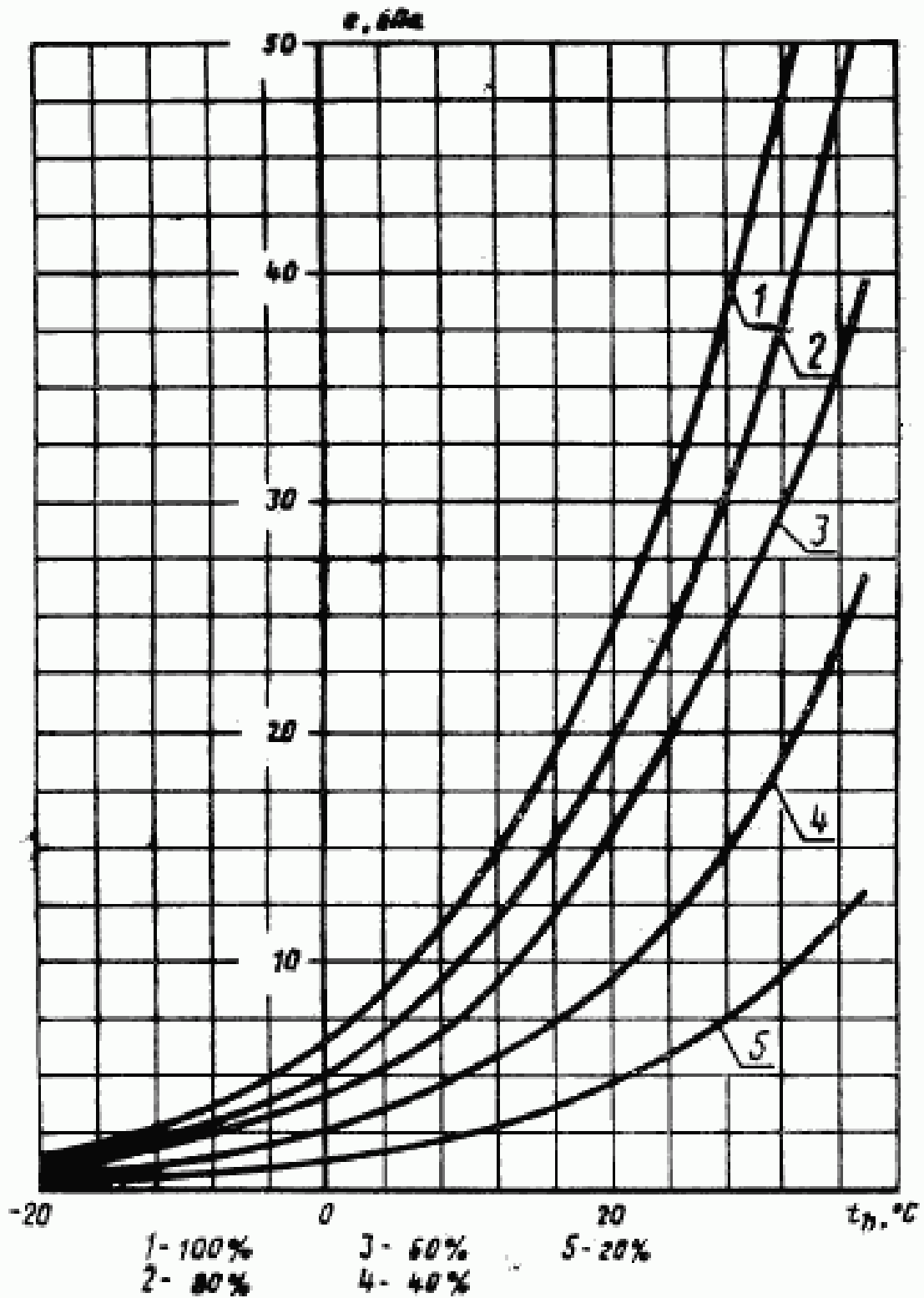
Номограмма зависимости парциального давления водяного пара e , относительной влажности воздуха U и температуры t_n
