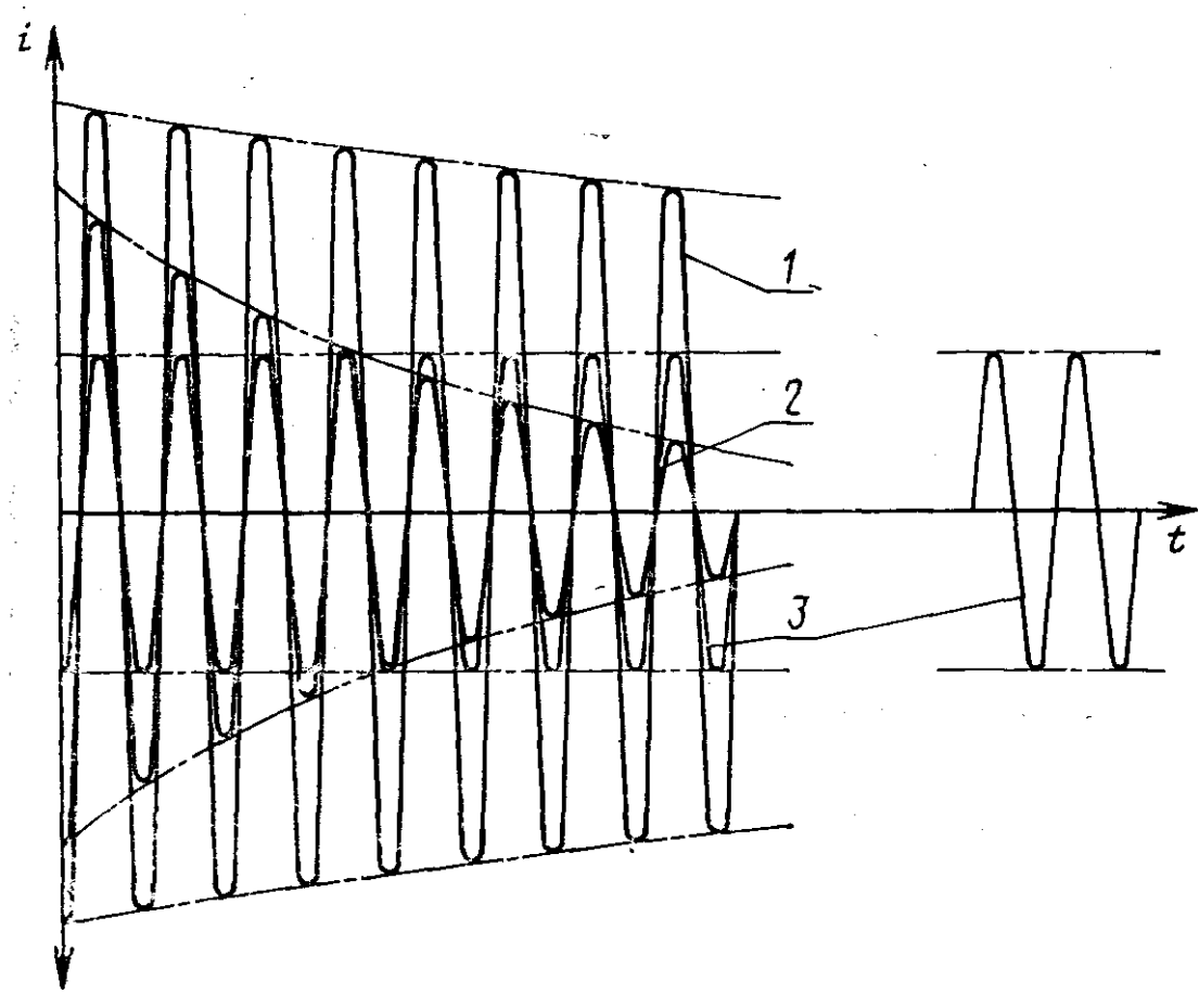
1—свободная переходная составляющая; 2—свободная сверхпереходная составляющая; 3—принужденная составляющая
