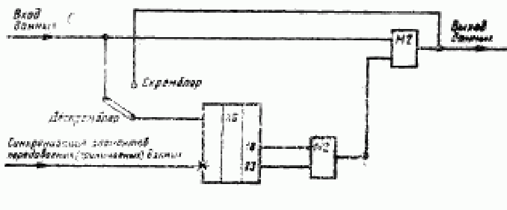
Функциональная схема скремблера-дескремблера для УПС-9,6 ТЧ
