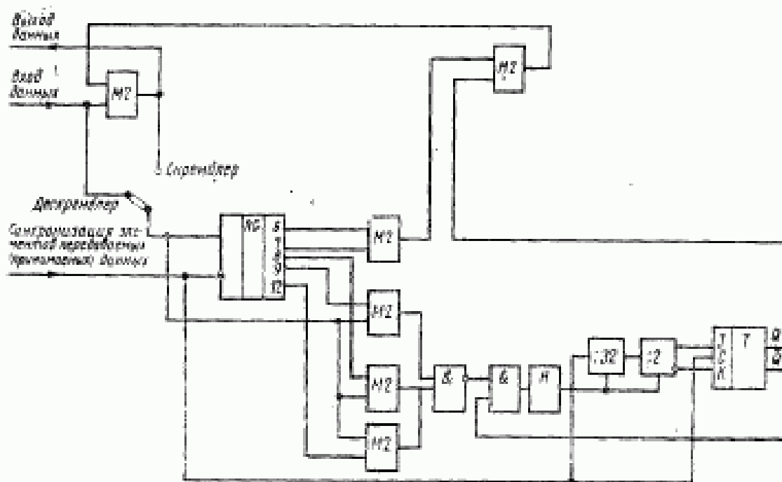
Функциональная схема скремблера-дескремблера для УПС-4,8 ТЧ
