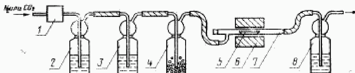
Схема установки для пиролиза
