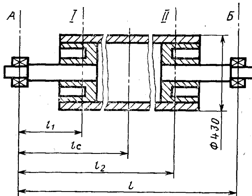
Схема расположения плоскостей коррекции вала
