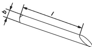
Рисунок А.7 — Копьевидный щуп
