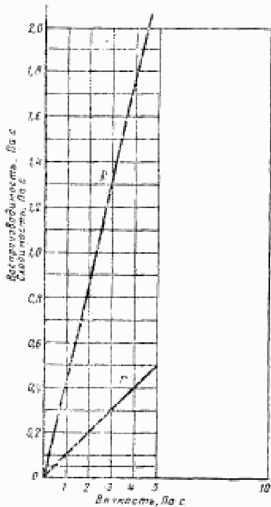
Зависимость показателей точности от вязкости до 5 Па·с
