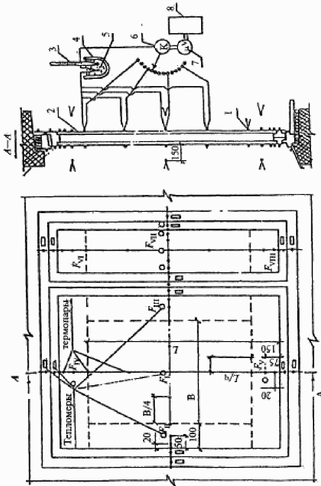
1 — рабочий слай термопары; 2 — испытываемый образец; 3 — термометр; 4 — сосуд Дьюара; 5 — холодный слай; 6 — многополюсный переключатель; 7 — микровольтметр; 8 — блок обработки и регистрации данных; F_I - F_{VIII} — термические однородные зоны
