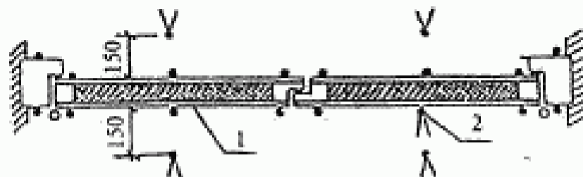
Рисунок 3 — Схема размещения термопар и тепломеров на образце дверного блока
