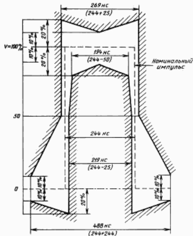
Вид и форма импульса кодированного сигнала
