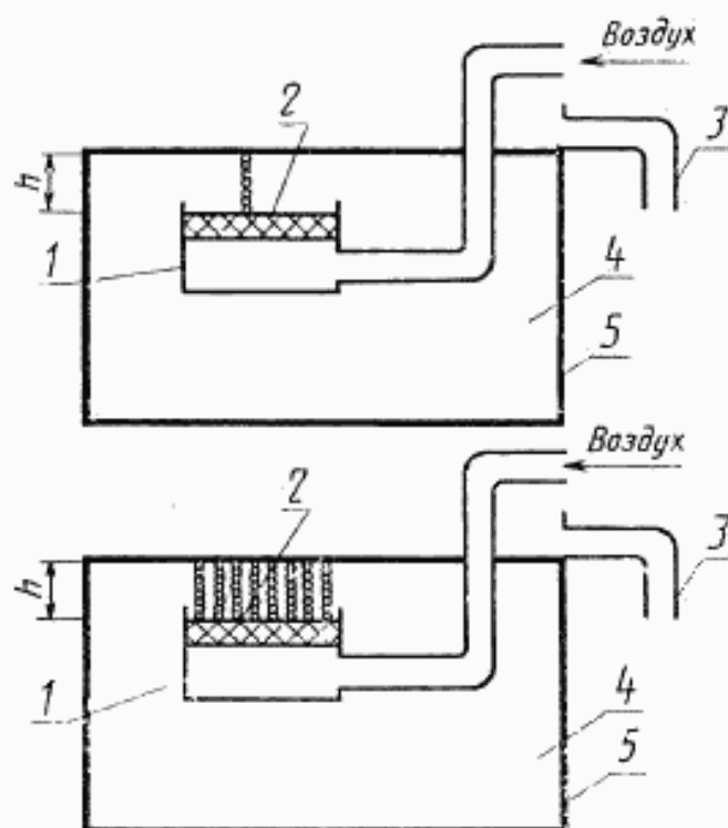
1—держатель образца; 2—испытуемый образец; 3—трубки для слива жидкости; 4—жидкость; 5—сосуд для жидкости; h —высота столба жидкости над испытуемым образцом.
