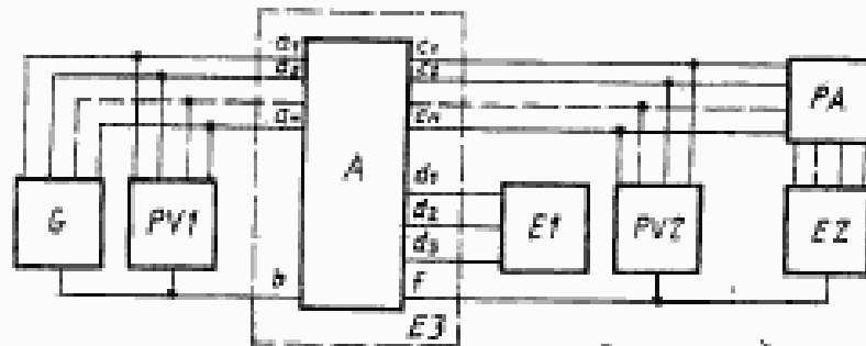
G —источник постоянного напряжения; PV1 —измеритель постоянного напряжения; A —НСН; a_1, a_2, \dots, a_n, b —входы НСН; c_1, c_2, \dots, c_m, f —выходы НСН; E1 —блок делителей; PV2 —измеритель постоянного напряжения; PA —измеритель постоянного тока; E2 —блок нагрузок НСН; E3 —устройство задания температурного режима; d_1, d_2, d_3 —выходы подключения обратной связи
