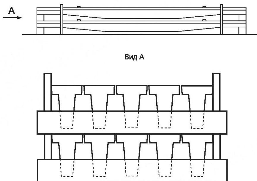
Рисунок 2 — Пример складирования прогонов таврового сечения
